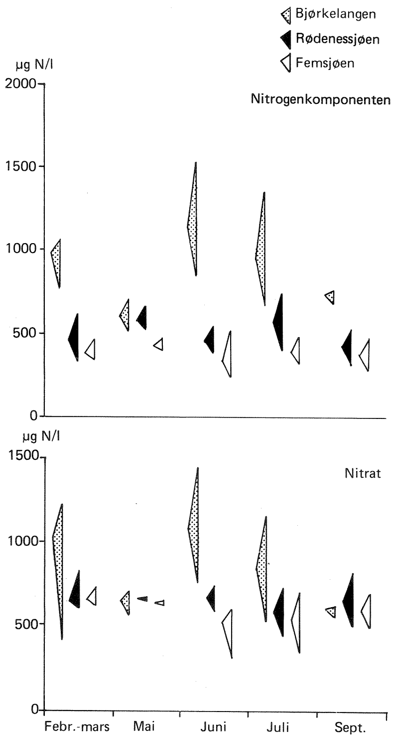
Fig. 13. Min., maks. og aritmetisk middelværdi for nitrogenkomponenter og nitrat i tiden febr. – sept. 1980.
