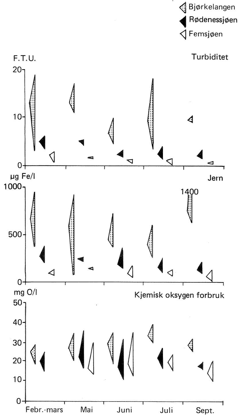
Fig. 11. Min., maks. og aritmetisk middelværdi for turbiditet, jern og kemisk oxygenforbrug i tiden feb. – sept. 1980.
