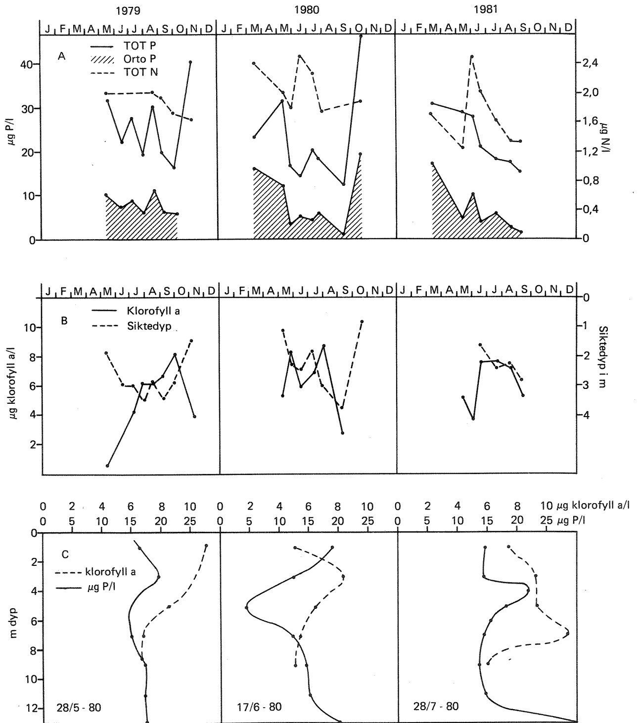
Fig. 7. Variasjon i midlere næringssaltinnhold (a), midlere klorofyll a og siktedyp (b) og vertikal fosfor- og klorofyllvariasjon på utvalgte observasjonsdager.
