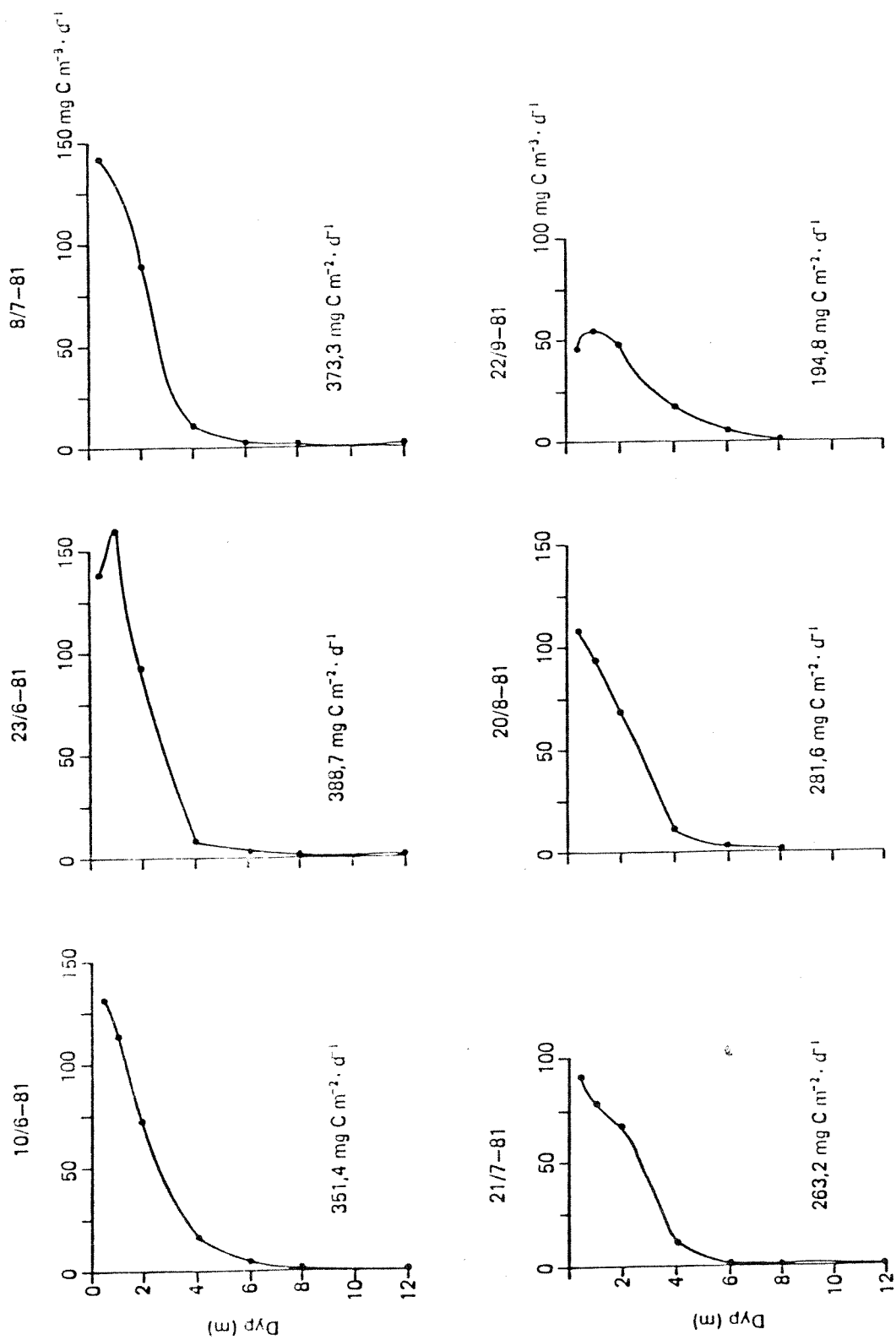
Figur 14. Utviklingen i algebiosmassens primærproduksjon i Øyeren gjennom perioden juni-september 1981.
