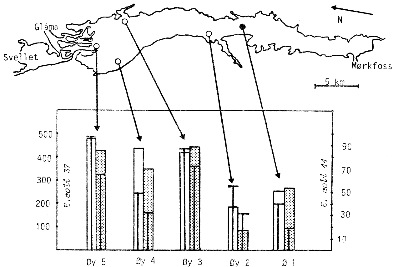
Figur 10. Grafisk fremstilling av middelverdiene for de bakteriologiske prøvene i 1980 og 1981 (T). Prøvene er tatt i overflatelaget i perioden juni-september (5 prøver). Åpne søyler angir koliforme bakterier ved 37 °C og skraverte angir termotolerante koliforme bakterier ved 44 °C. Verdiene er antall pr. 100 ml.
