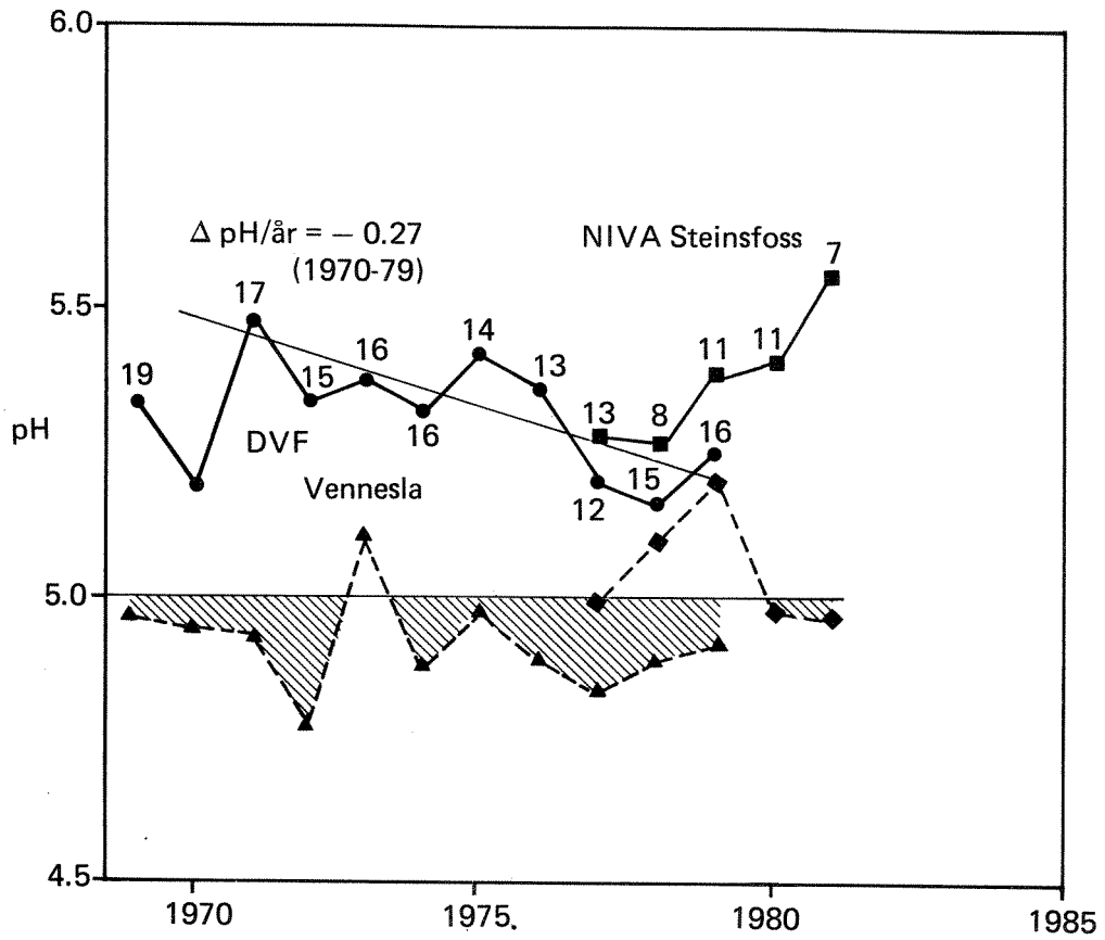
Figur 6: Arsmiddel pH og minimum pH målt over perioden 1969-1981 i Otra ved Vennesla og Steinsfoss. Antall prøver er angitt. Otra er fra DVF's elveserie (sirkler) og NIVA (firkanter overvåking). Regresjonslinje er fra Henriksen et al. (1981).
