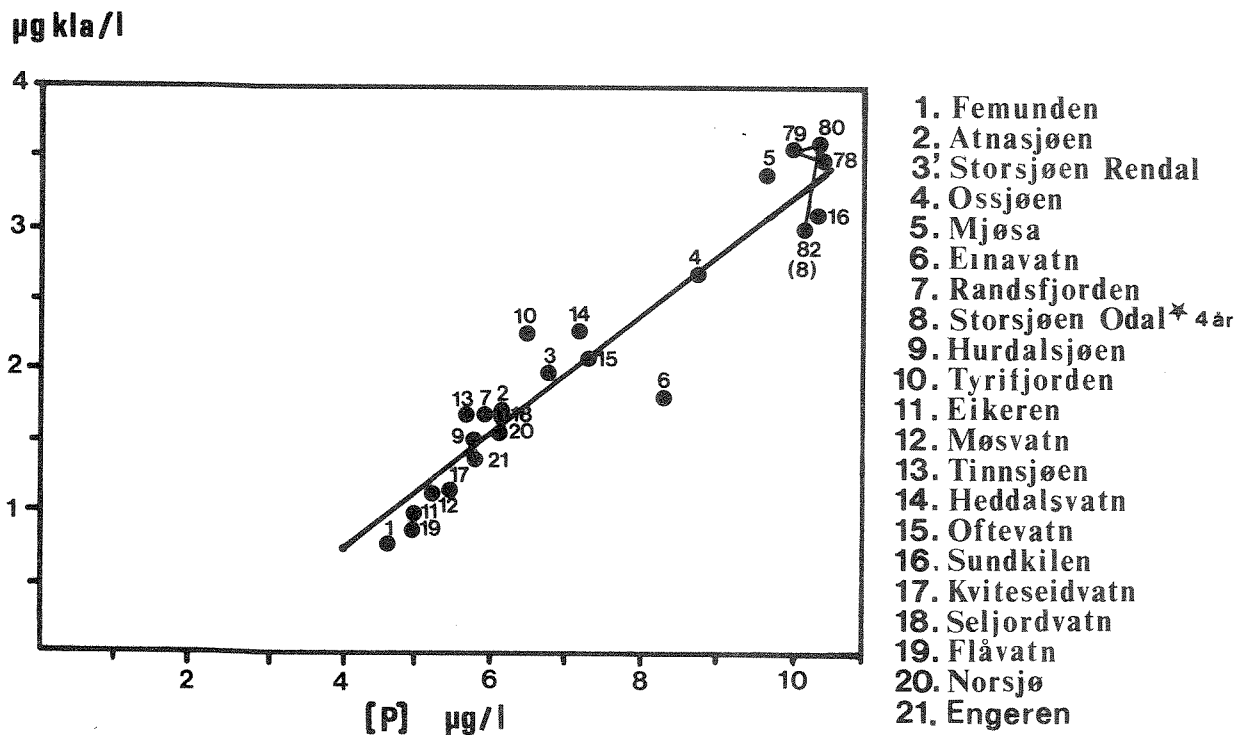
Fig. 16. Sammenhengen mellom middelkonsentrasjon av fosfor og gjennomsnittlig algemengde (som klorofyll a) i epilimnion for flere norske innsjøer.
