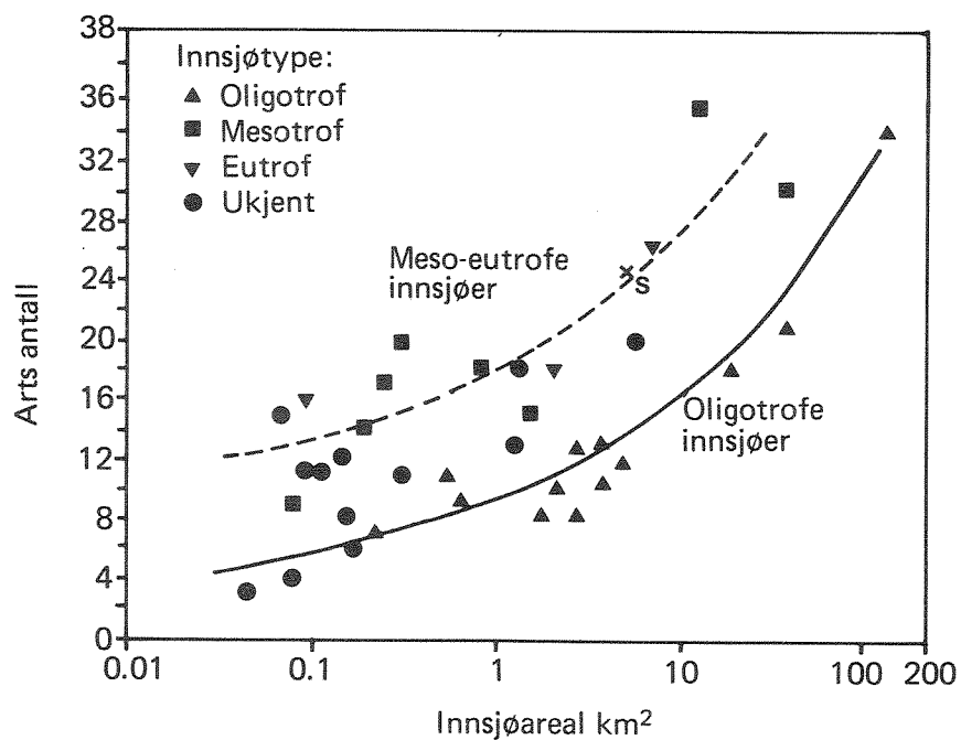
Fig. 7.7. Sambandet mellom innsjø-areal og artsantall (gruppene elodeider, isoetider, lemnider og nymphaeider) i endel norske innsjøer. S=Svullet. Modifisert etter Rørslett 1983.
