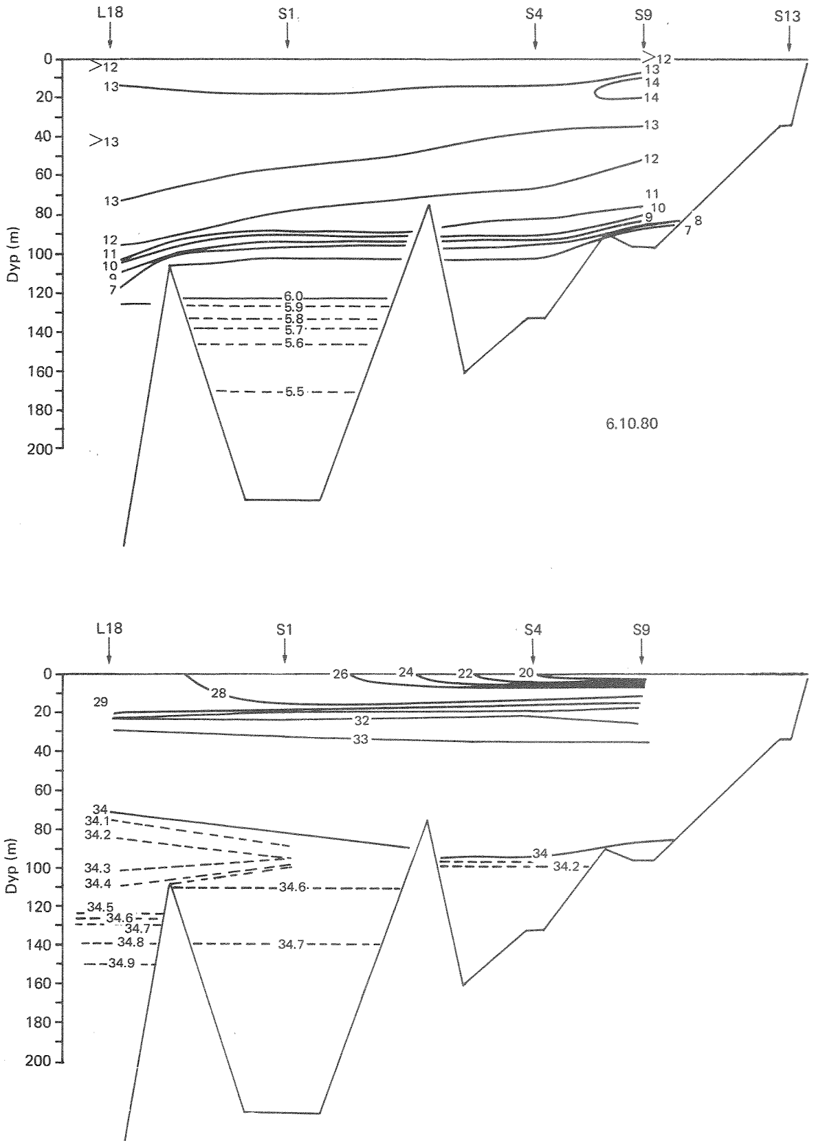
Fig. 6.2 Temperatur (øverst) og saltholdighet (nederst) i Kosterfjorden-Singlefjorden 6.10.80.
