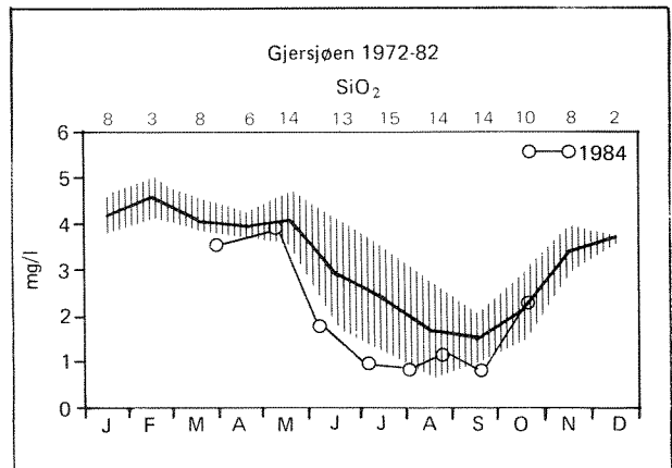
Figur 6.7 Silikat
