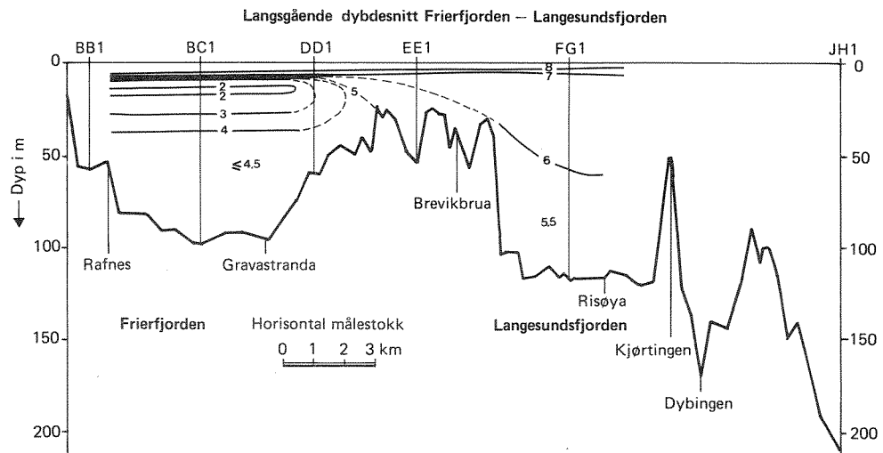
Figur 4.2 Oksygenkonsentrasjoner (ml O 2 /l) i Friierfjorden og Langesundfjorden 4. mai 1984.
