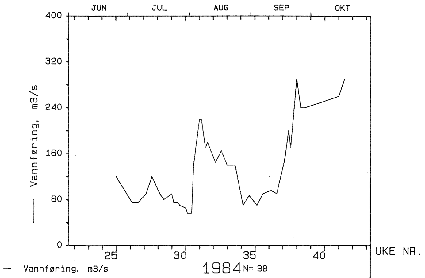
Figur 2.2 Vannføring ved Skotfoss 1984 på dager med laksetelling.
