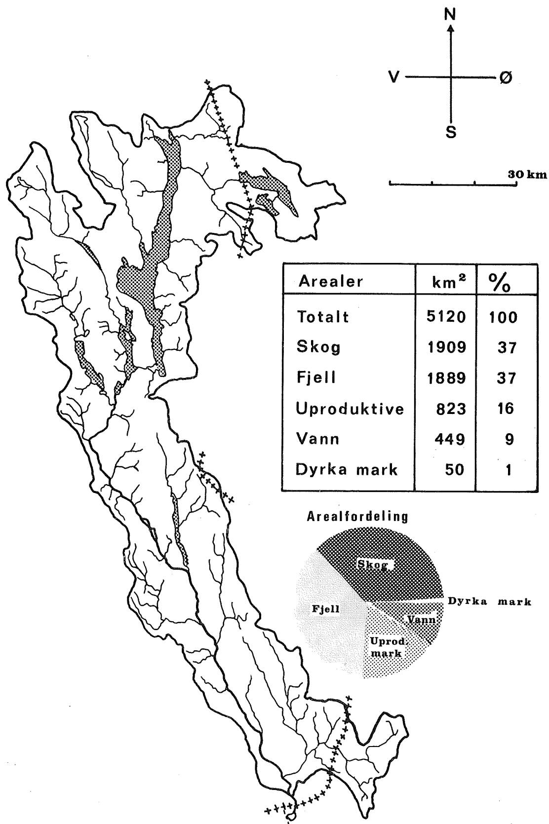
Figur 2. Trysilelvas nedbørfelt.
