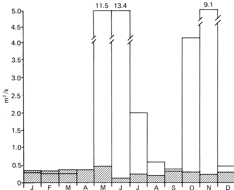
Figur 2. Eks. på avrenning fra Finnfjordvatn og Industriområdets vannbehov (år 1978). Hydroconsult 1985. En årlig middelvannføring på 3,28 m^2/s blir lagt til grunn for avrenningen (skravert = vannbehov).
