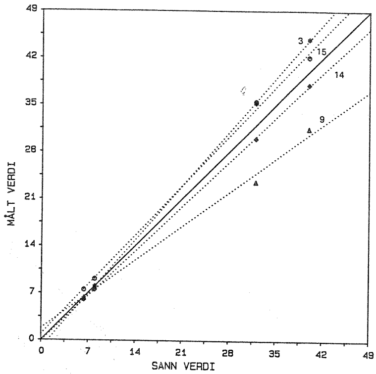
FIGUR 12. "KALIBRERINGSKURVER"
