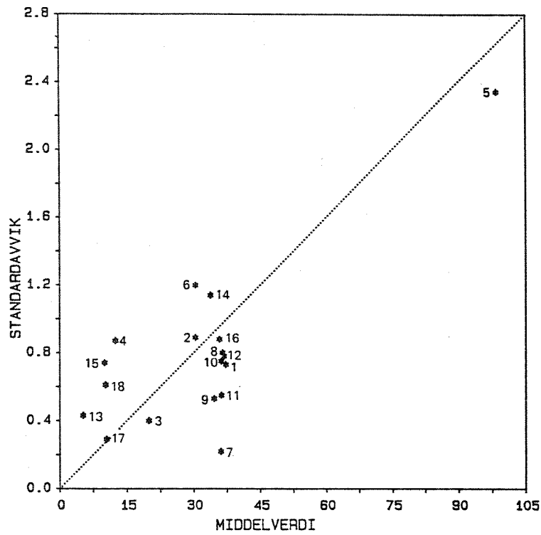
FIGUR 14. INTERNKONTROLLRESULTATER
