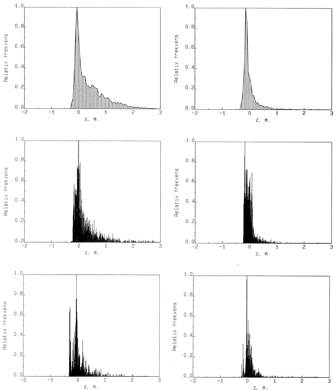
Fig. 2. Fordeling av beregnede vannstander, z , i Venneslafjorden, fra likn. (2) med b=1 . Fordelt på hhv. sommer (venstre) og vinter (høyre) for åra 1930-1950 (øverst), 1964-1979 (midt) og 1980-1985 (nederst). Vannstand angitt som avvik fra medianvannstand (kote 38.18-38.27, jfr. tab. 2). Negative verdier er under, positive verdier over medianvannstand. Jfr. tekst for usikkerhet i beregnet høy vannstand ( z \approx +1 og større). Sommer: uke nr. 17-40 Vinter: uke nr. 1-16, 48-52. Basert på døgnmålinger ved VM 1007 Vigeland.
