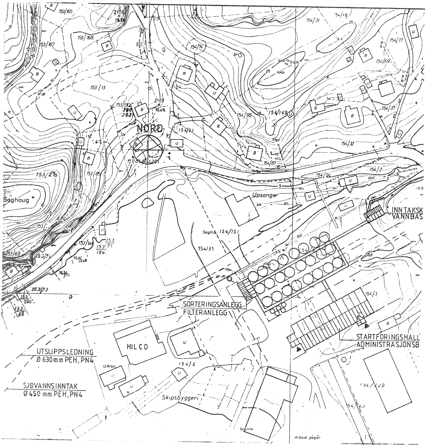
Fig. 3. Opsangervågen. Setjefiskanlegg. Forskingsbygg.
