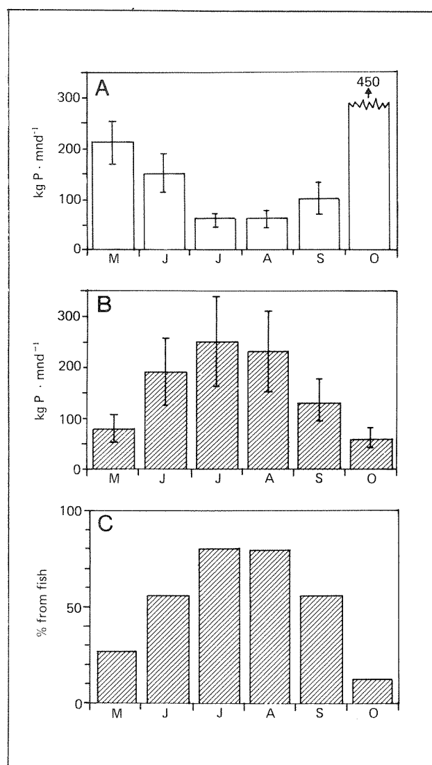
Figur 6.22 Målt tilførsel av fosfor fra Gjersjøens tilløpsbekker 1980 og beregnet bidrag fra mort (fra Brabrand og medarb., under utarb.) Det er antatt omtrent samme mengde fisk i innsjøen hele året ved denne beregningen. A: Fra nedbørfeltet B: Fra mort C: Prosentandel fra mort
