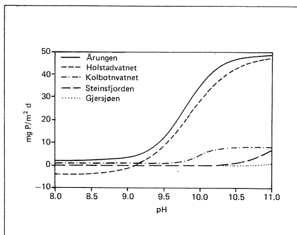
Figur 6.23 Fosfat kan frigjøres i store mengder fra grunnvannsedimenter i enkelte innsjøer på Østlandet, men har neppe betydning i Gjersjøen (etter Sanni 1984 og denne undersøkelse).
