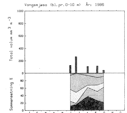
Fig.10 Variasjon i totalvolum og sammensetning av planteplankton i de undersøkte innsjøene i Begnavassdraget 1984-86. Blandprøver 0-10 m.
