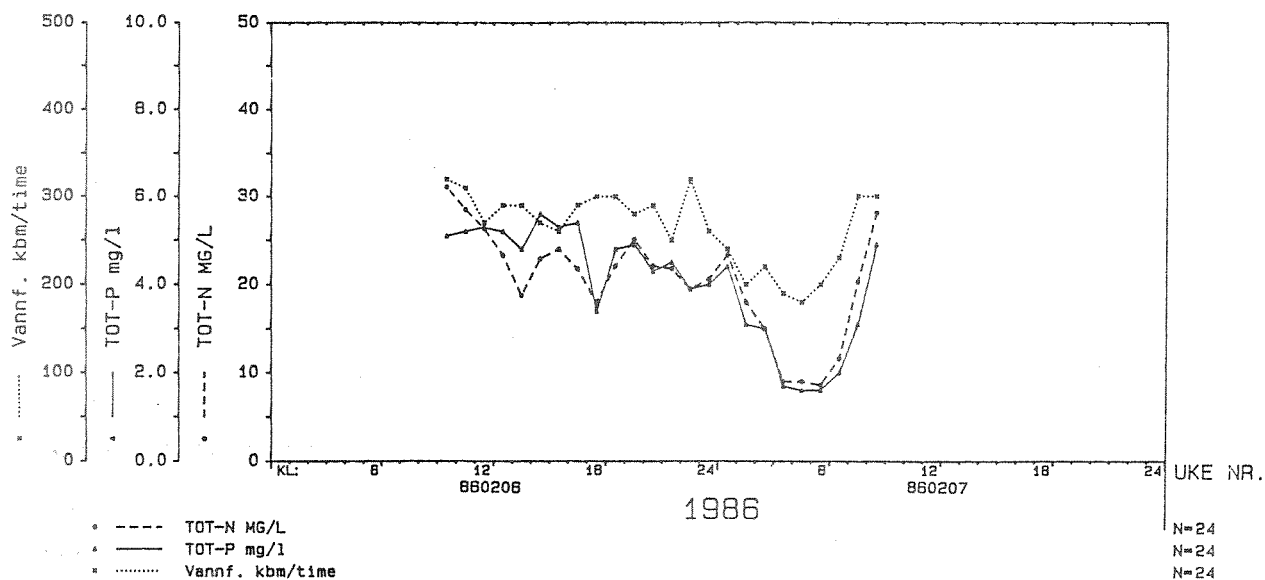
Figur 10. Forurensningskonsentrasjoner i Holmen-påslippet.
