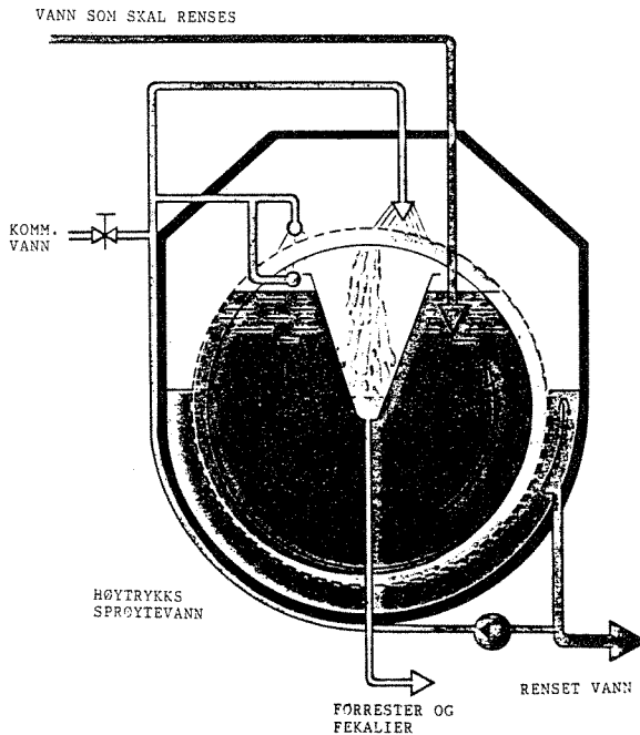
Figur 1. Prinsippskisse av Algas Microfilter.
