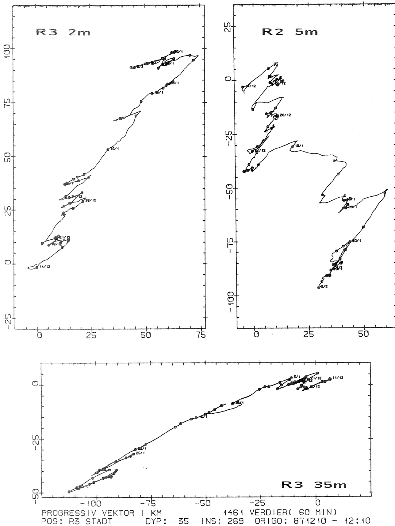
Fig. 4.4. Progressive vektordiagram for strømmålingene på R3, samt R2 i 5 m, med ytre terskelen til Kjødpollen.
