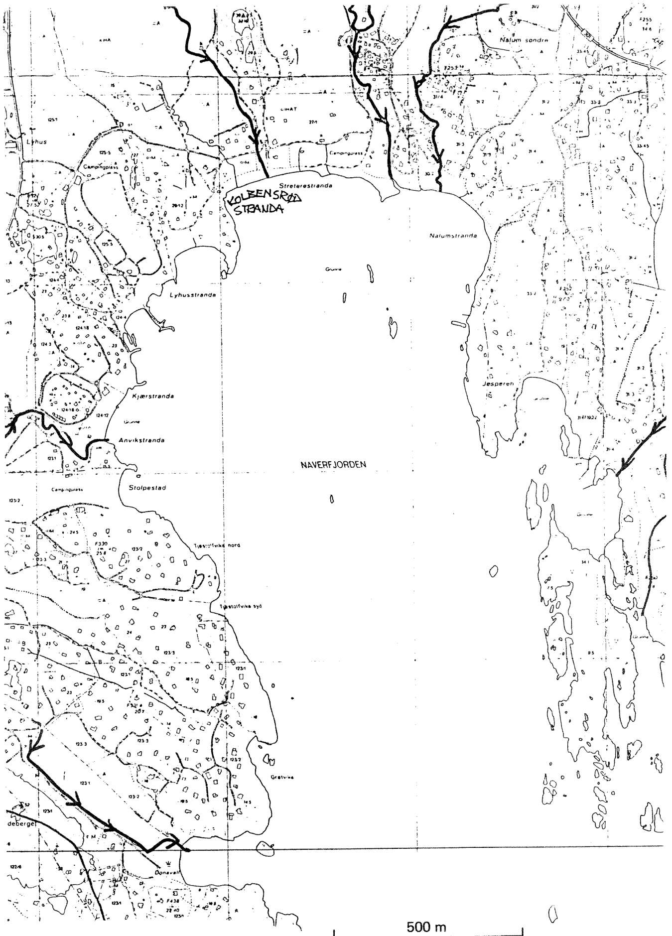
Fig. 15. Naverfjorden med hovedvassdragene (bekken) inntegnet.
