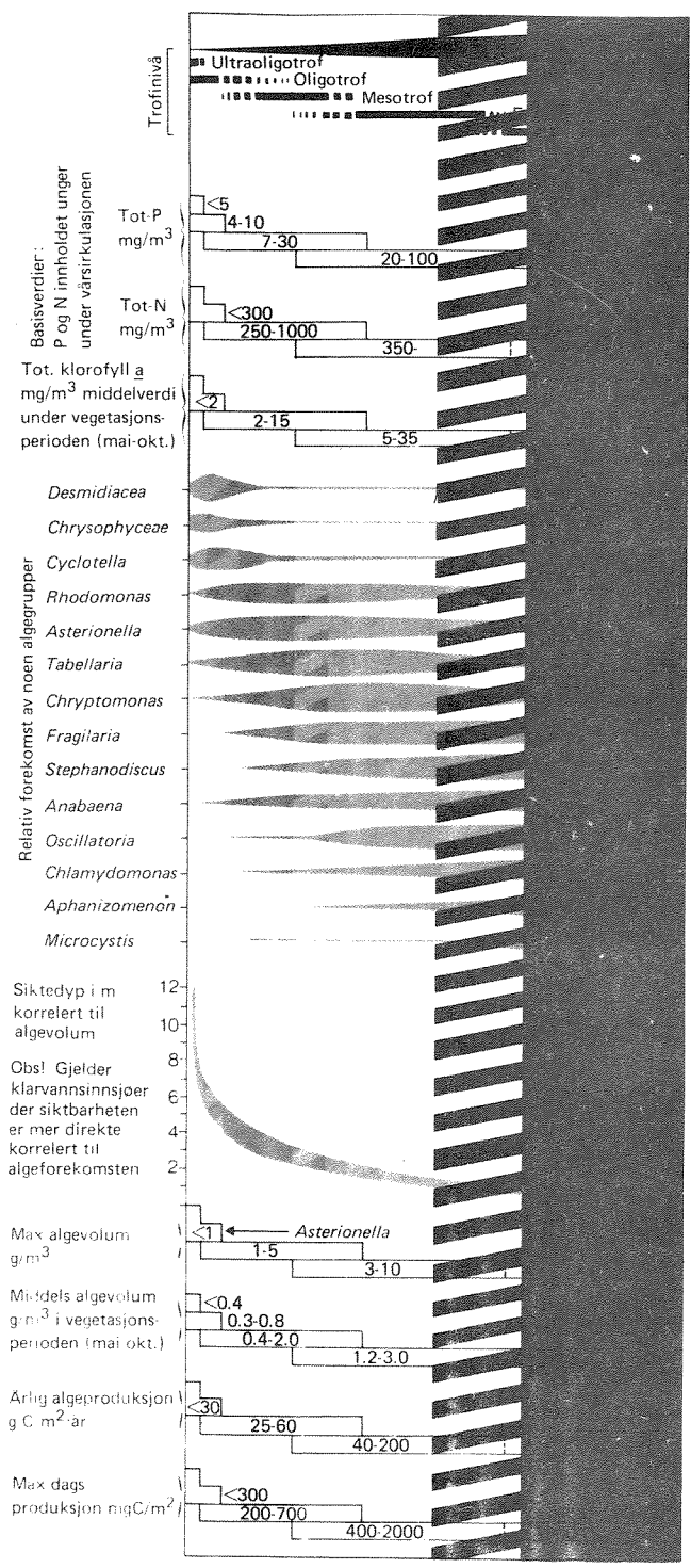
Fig. 18 Vollenweiders eutrofimodeller (1968, 1976) og det såkalte »miljøregel» er gode redskap når det gjelder å bedømme belastning - respons i store og dype innsjøer. Diagrammet har dog sin klare begrensning og må anvendes med varsomhet.
