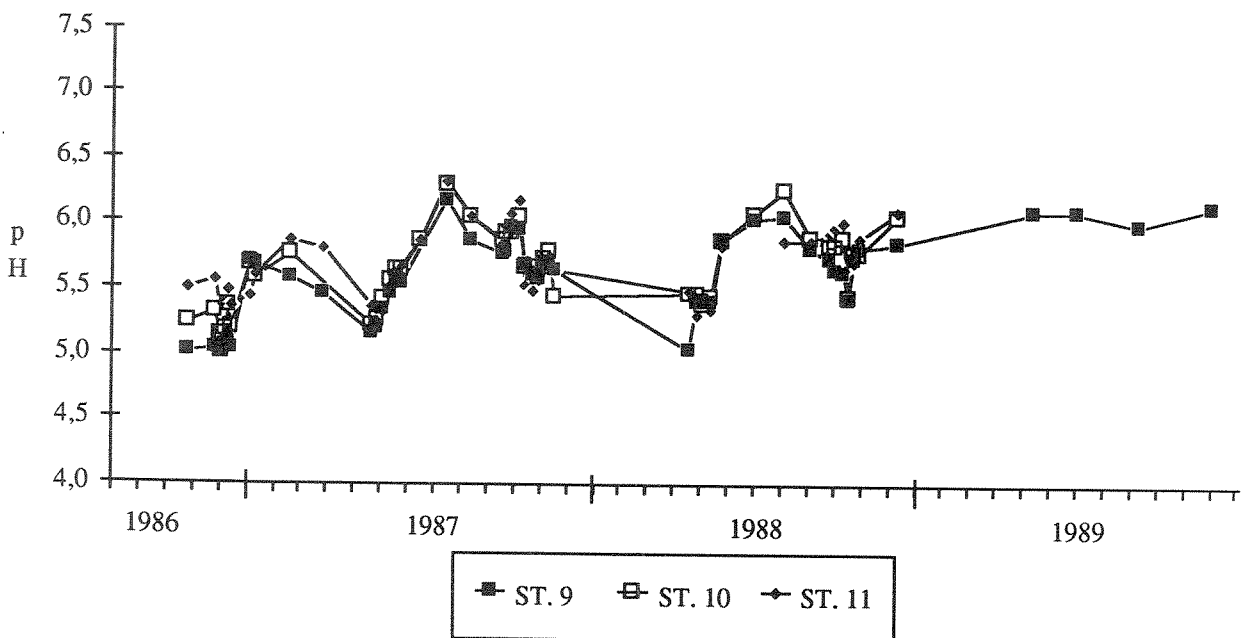
Figur 4. pH i Vegårvasselvea oppstrøms (St. 7) og nedstrøms (St. 8) kalking, utløp av Vegår (St. 9), Storelva ved Ubergsmoen (St. 10) og Storelva ved Nes Verk (St. 11) i perioden 1985-1989.
