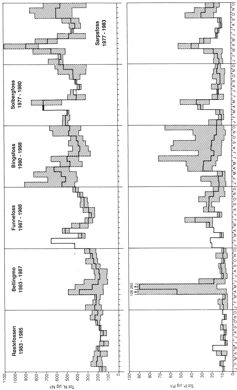
Fig. 8.6 Variasjon i konsentrasjoner av total nitrogen og total fosfor i løpet av året. Maks., min. og middel for månedsværdiene er tegnet inn.
