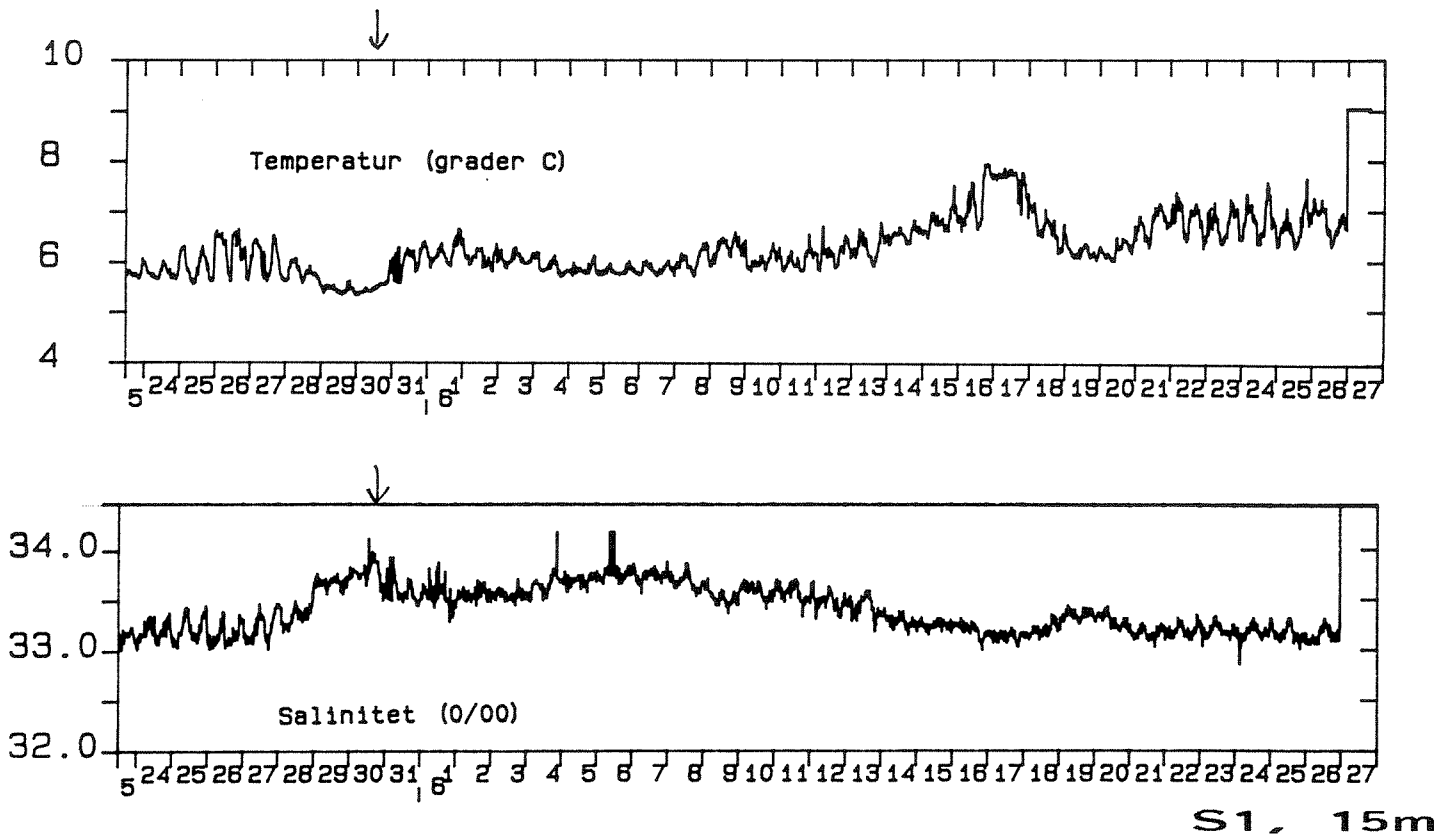
Figur A27. Målt temperatur og salinitet på S1, 3 m dyp og 15 m dyp perioden 23/5-6/6. Riggeren havarerte 30/5.
