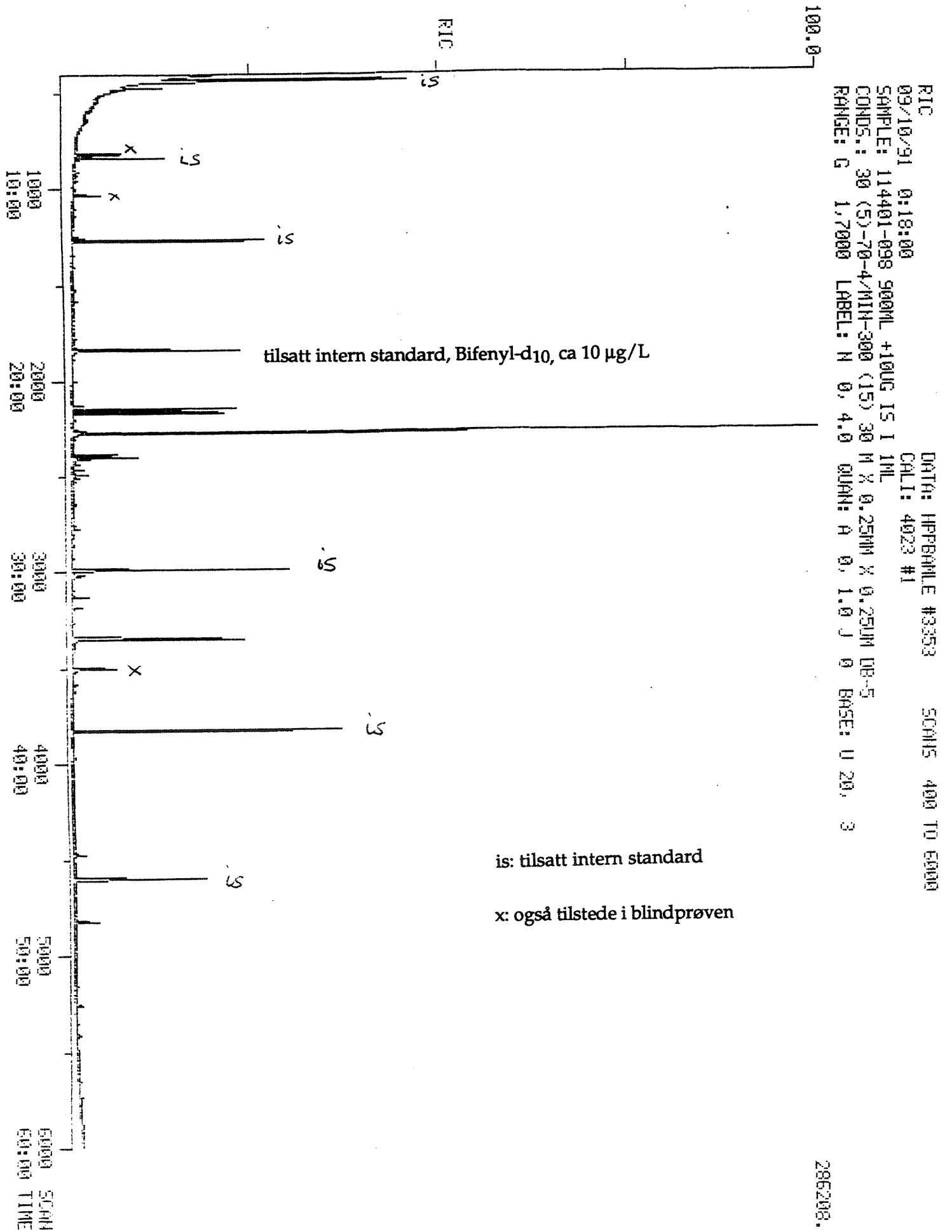
Figur 1. GC/MS-kromatogram av "Blandprøve, utløp renseanlegg 3-7/6-91"
