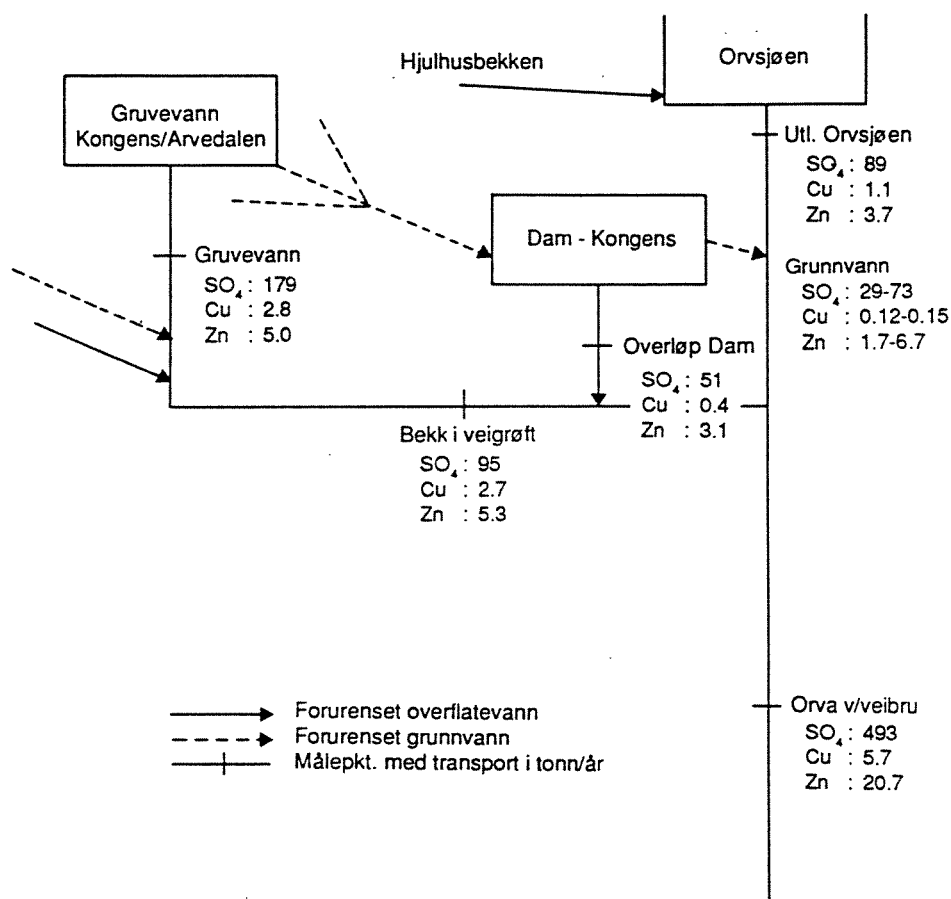
Figur 1. Skjematisert fremstilling av forurensningstransport i Nordgruvefeltet, 1990 Alle mengdeangivelser i tonn/år. (Etter Arnesen 1991a)
