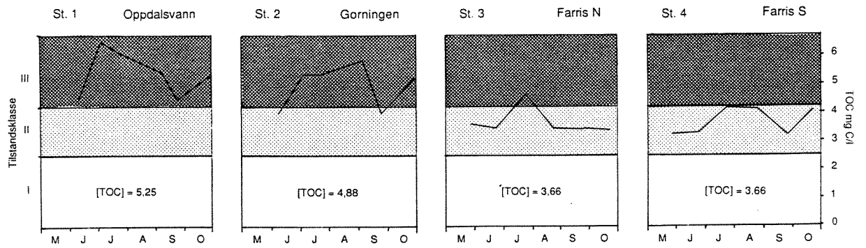
Fig 5.7 Overflate blandprøve. Variasjon i total organisk karbon (TOC). [TOC] = veide middelveier i mg C/l.
