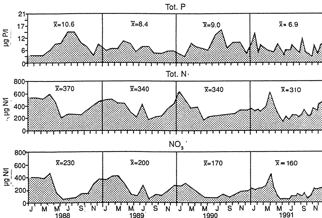
Fig.21 Månedlige middelværdier for konsentrasjonen av næringssalter i Dokka (Kolbjørnshus) i perioden 1988-91.
