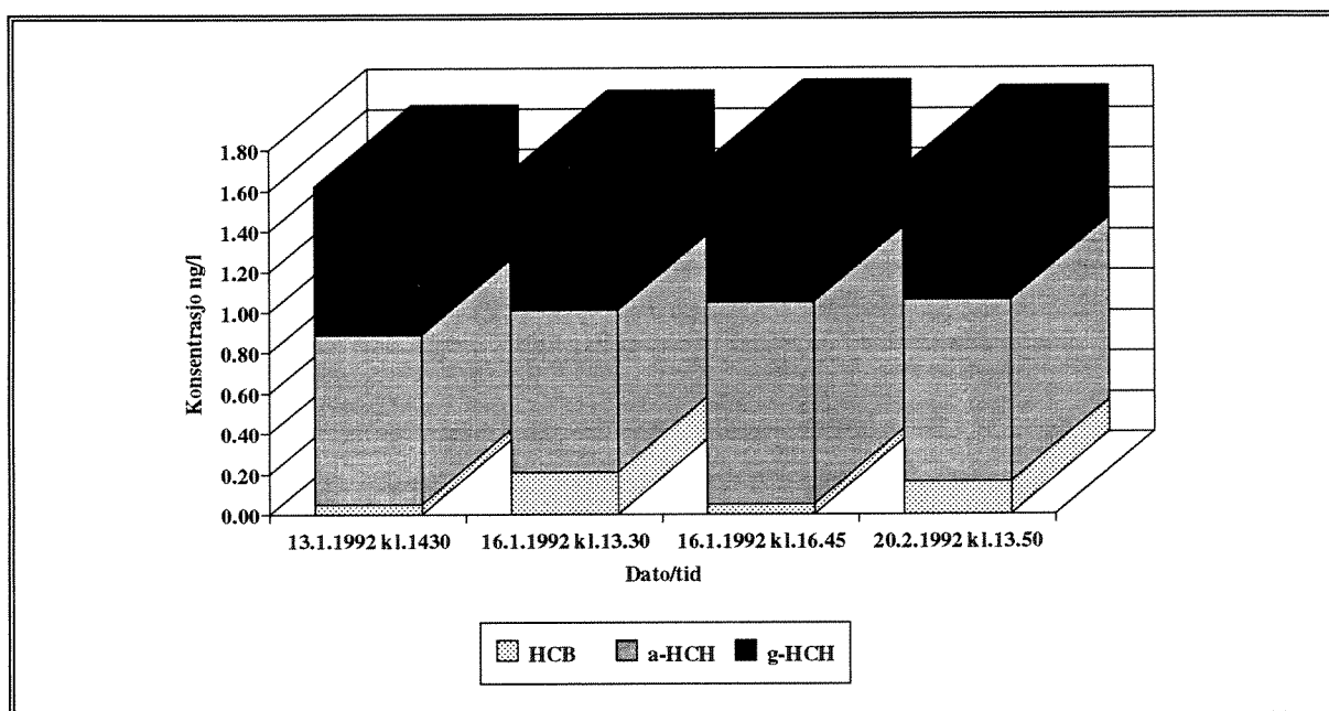
Figur 9. Konsentrasjoner i ng/l av HCB, \alpha -HCH (heksaklorsyκλοheksan) og \gamma -HCH (Lindan) målt i 23 m vanddyp på stasjon III, Kristiansandsfjorden i perioden 13.01-20.02.1992.
