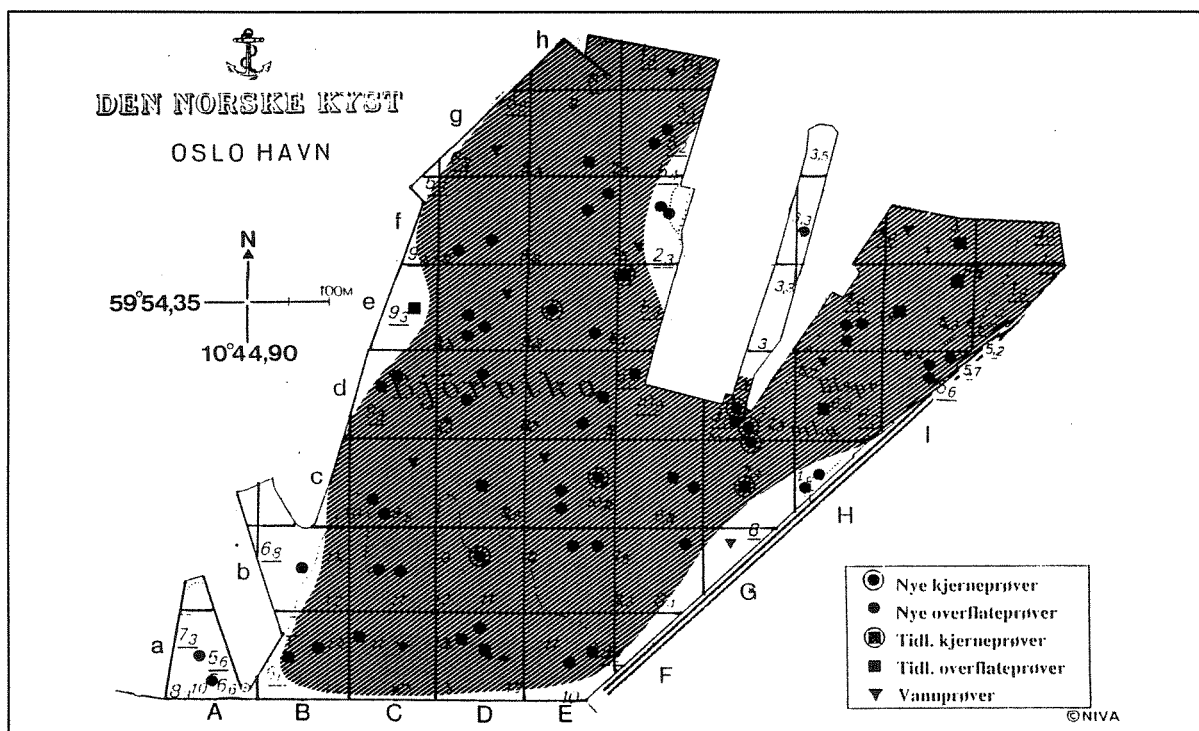
Figur 7. Horizontalutbredelse av markert eller sterkt forurensede overflatesedimenter (0-2cm) med hensyn på kobber (>150 mgCu/kg tørt sediment, >4x overkonsentrasjon).
