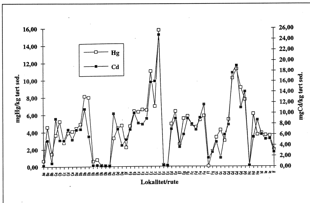
Figur 2. Konsentrasjoner av Hg og Cd i mg/kg tørt sediment målt i bunnsedimentene i området Bjørvika - Bispevika, Oslo havn.
