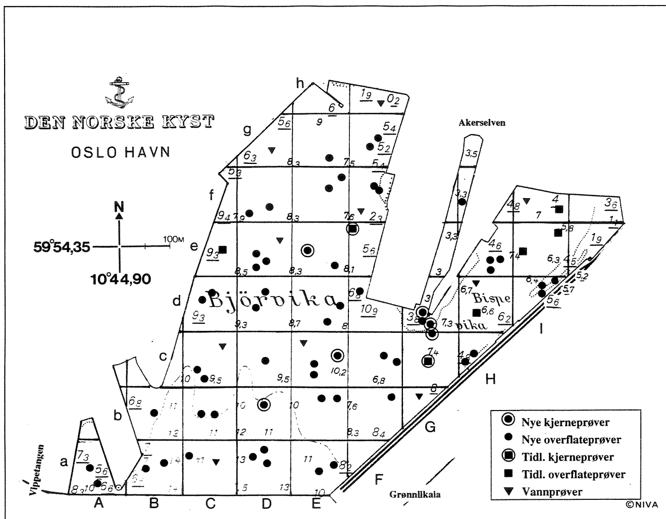
Figur 1. Kart over undersøkelsesområdet Björvika - Bispevika, Oslo havn, med fullstendig prøvedekning avmerket (inkludert tidligere rapporterte stasjoner). Det inntegnede rutenett har målestokk 100x100m.
