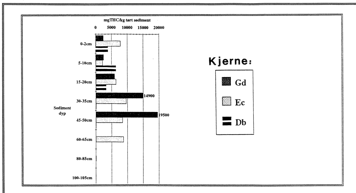
Figur 13. Vertikal forekomst av THC i mg/kg tørt sediment i tre kjerne sentralt i området Bjørvika - Bispevika, Oslo havn.
