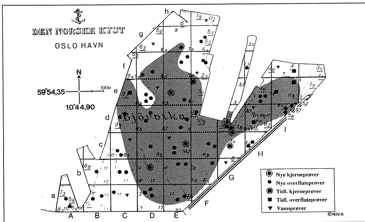
Figur 5. Horizontalutbredelse av sterkt forurensete overflatesedimenter (0-2cm) med hensyn på kadmium (>5 mgCd/kg tørt sediment, 20x overkonsentrasjon).
