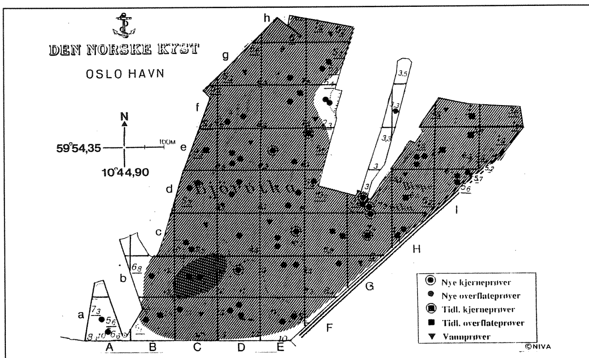
Figur 6. Horizontalutbredelse av markert og sterkt forurensete overflatesedimenter (0-2cm) med hensyn på bly (>120 mgPb/kg tørt sediment, >4x overkonsentrasjon).
