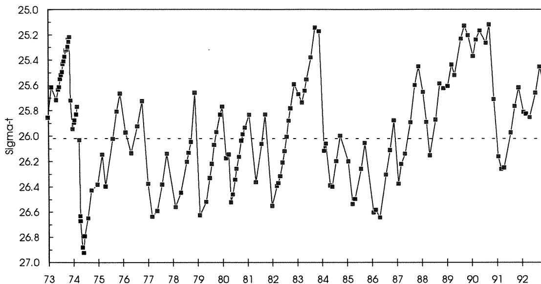
Figur 28. Egenvekten (sigma-t) på 80 meters dyp i Vestfjorden 1973-92. (Stiplet linje viser middelværdi for perioden).
