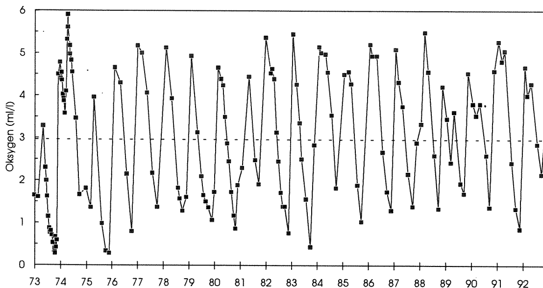
Figur 25. Oksygenkonsentrasjonen på 80 meters dyp i Vestfjorden (Dk1) 1973-82. (Stiplet linje viser middelerdi for perioden).
