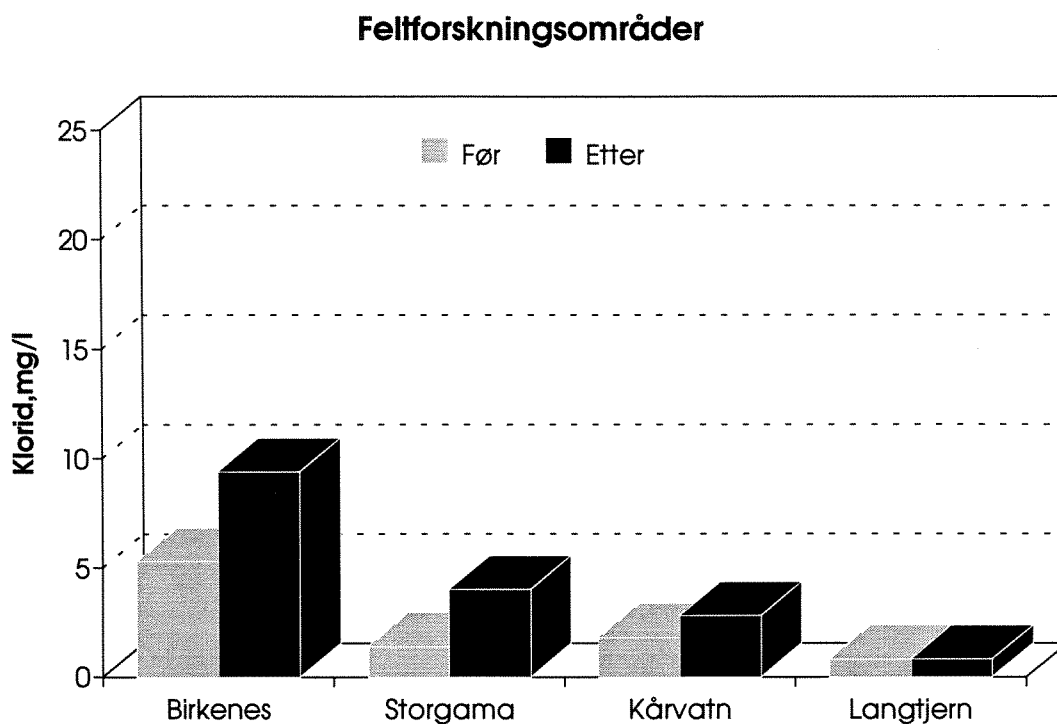
Figur 15. Kloridkonsentrasjoner i feltforskningsområder. Dataene er fra programmet for overvåking av langtransportert forurenset luft og nedbør (SFT).
