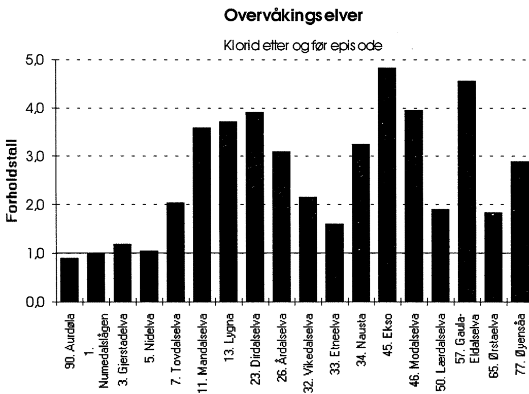
Figur 16. Forholdstall for kloridkonsentrasjonene etter og før sjøsaltepisoden for overvåkingselver.
