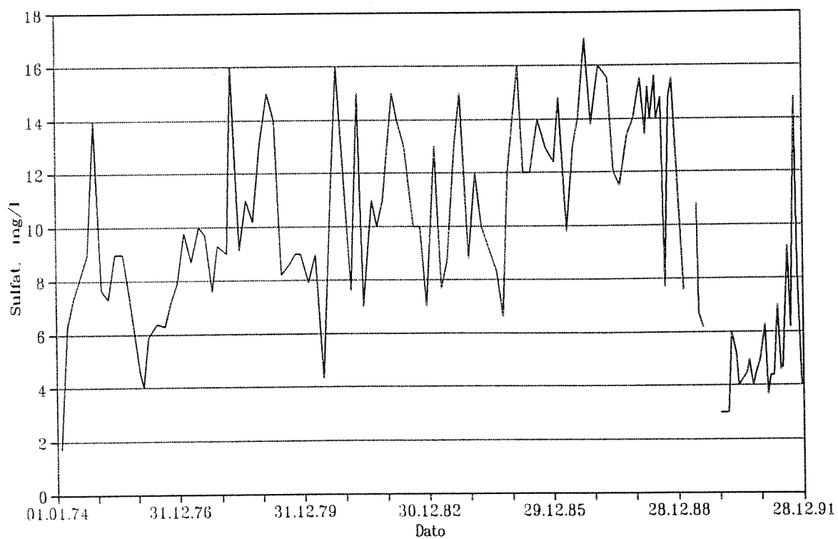
Figur 3.3.4 Analyseresultater fra Huddingselva (H8). Enkeltverdier - sulfat-konentrasjon.
