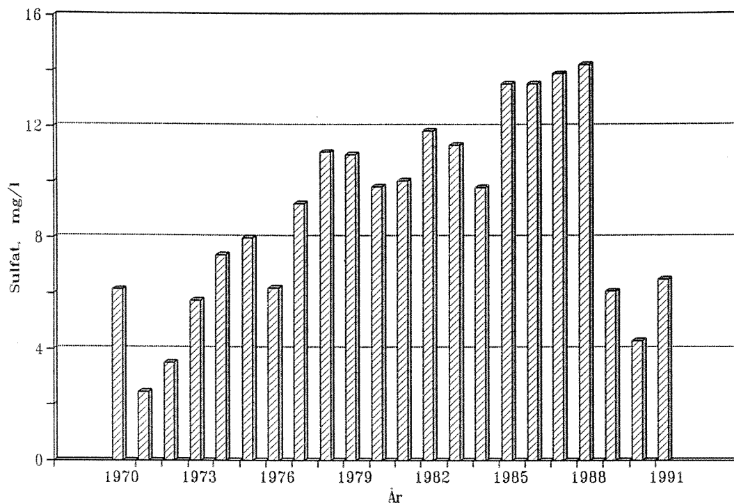
Figur 3.3.6 Tidsveiet årsmiddel for sulfat - konsentrasjon i Huddingselva (H8).
