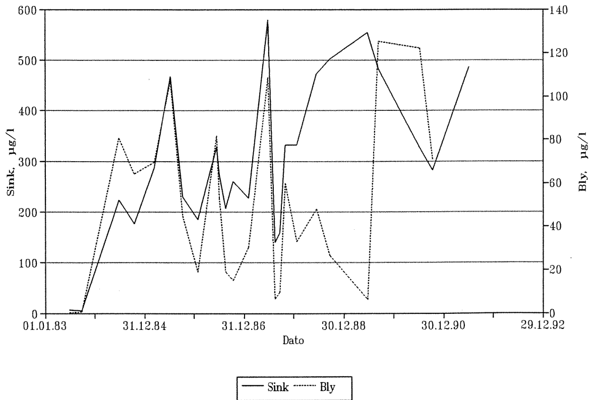
Figur 3.5.11 Middelkonsentrasjon av sink og bly ved B6, Kjøkkenbukta i Store Bleikevatn 1983 - 1991
