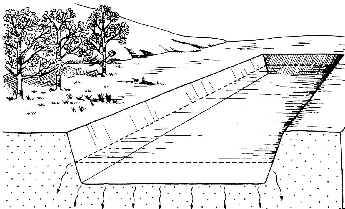
Prinsippskisse av et åpent infiltrasjonsbasseng.
