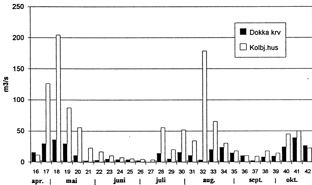
Figur 4. Vannføring (ukemidler) ved utløpet av Dokka kraftstasjon og Dokka/Etna (Kolbjørnshus).
