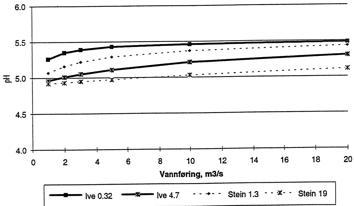
Figur 5. Resultat-pH etter blanding av vann fra Otravann med vann fra lokalfeltene Iveland og Steinsfoss. Vann fra Otravann er lagt inn med pH 5.5 i beregningene, mens vann fra lokalfeltene er lagt inn med pH 4.5 (øverst) og 4.9. Vannføringen i lokalfeltene er hhv. middelvannføring og antatt maksimal vannføring.
