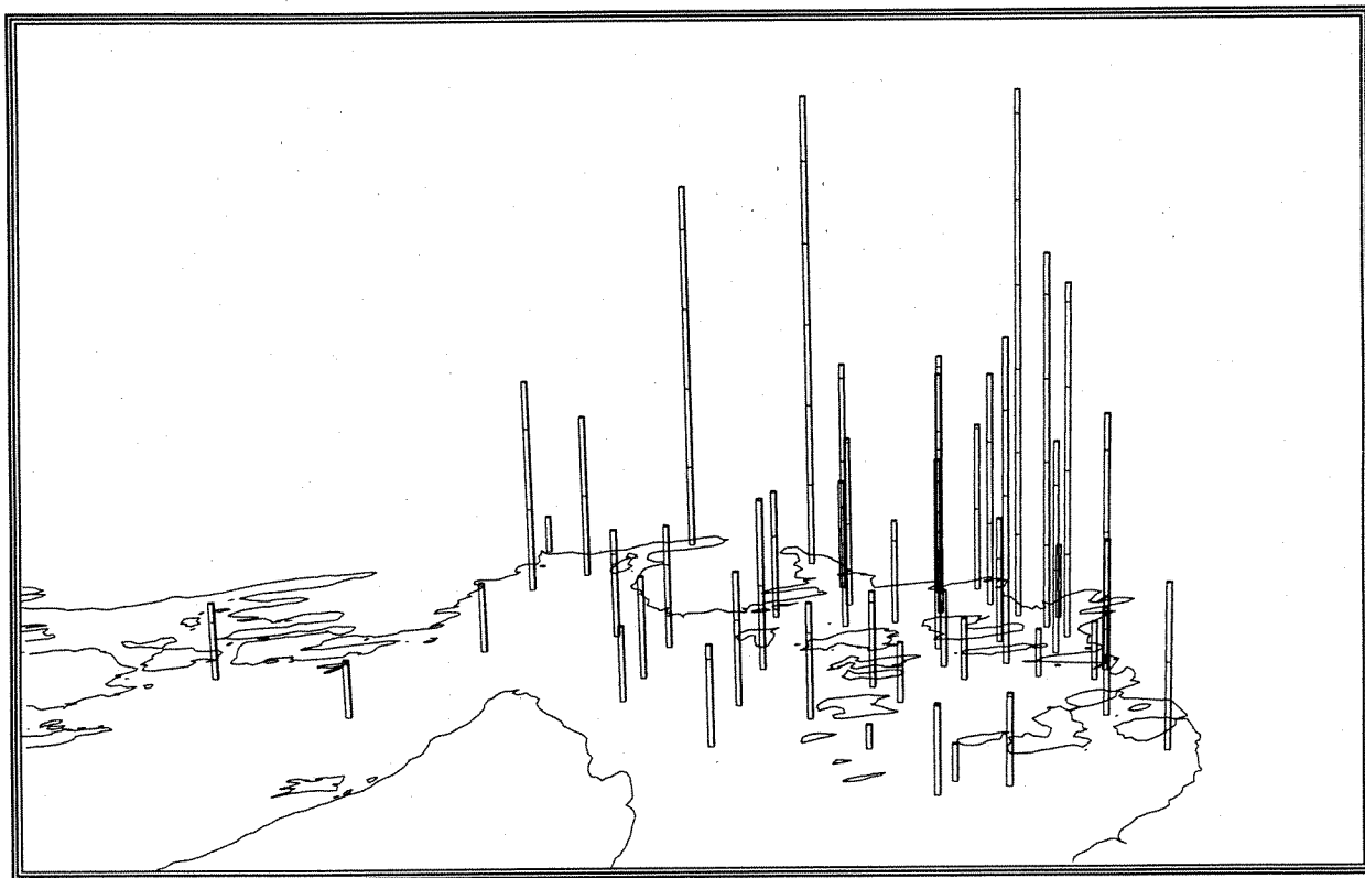
Figur 11. PCB forekomster i overflatesedimenter (1 delstrek = 100 µg/kg tørrvekt) i havnebassenget og Lysakerfjorden, Indre Oslofjord, 1992.
