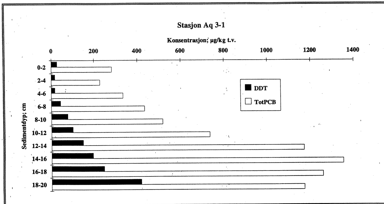
Figur 13. Vertikal forekomst (0-20 cm) av total PCB og sum DDT ( \mu\text{g}/\text{kg} tørrvekt) i sedimentene ved Akershuskaia, Indre Oslofjord 1992.
