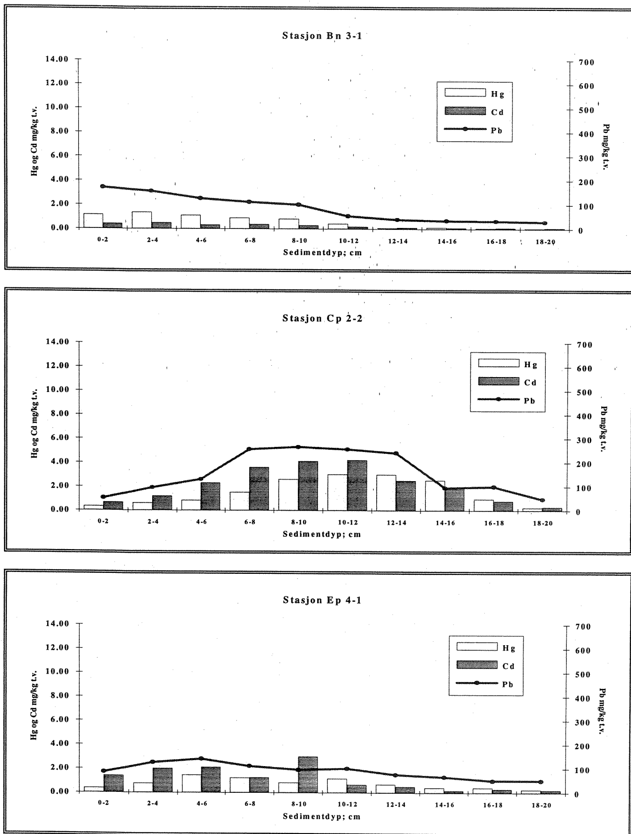
Figur 4. Vertikal forekomst (0-20 cm) av Hg, Cd og Pb (mg/kg tørrvekt) i sedimentene syd i hhv. Lysakerfjorden, Bekkelagsbassenget og Bunnefjorden, Indre Oslofjord 1992.
