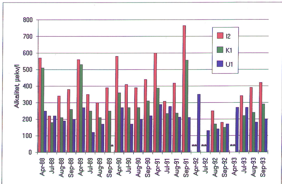
Figur 2.5. Sulfat (sjøsaltkorrigeret) og alkalitet i Tana's største sidevassdrag. I2: Anarjohka, K1: Karasjohka, U1: Utsjoki. * : ingen prøve.
