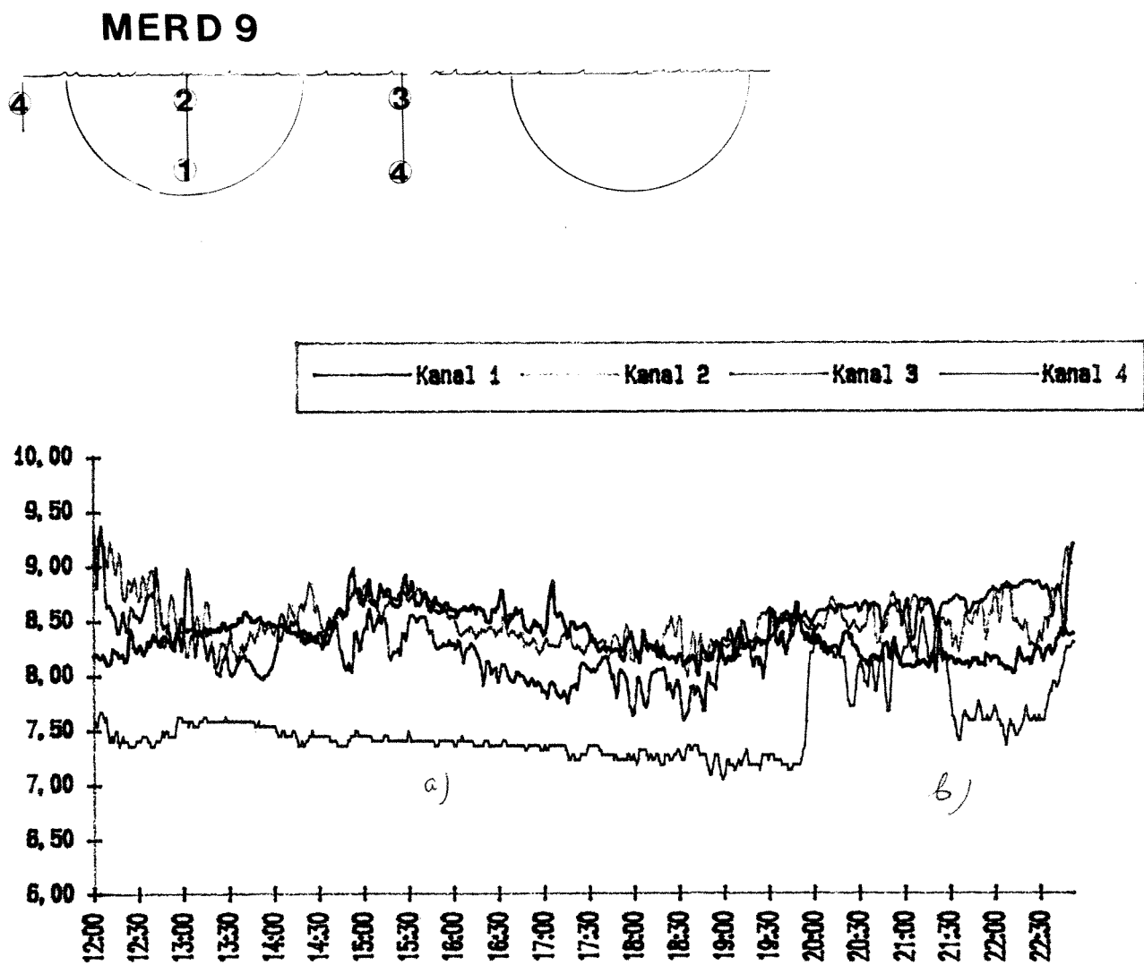
Figur 5. Oksygen i mg O 2 /l i merd 9 i perioden 22/6 - 94 kl: 11.50 - 23.00. Kanal 1 viser 10 m dyp midt i merden, kanal 2, 2 m dyp midt i merden, kanal 3, 2 m dyp utenfor merden (østside) og kanal 4, først 10 m dyp utenfor merd (østside) og deretter 2 m dyp utenfor merd (vestside).
