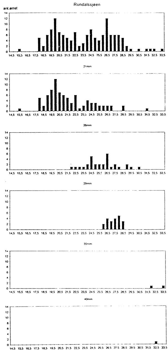
Fig.26 Lengdefordeling av abbor og ørret fanget ved prøvefiske i Rundalsjøen høsten 1993. Totalfangst og fangst pr. garnstørrelse er angitt.
