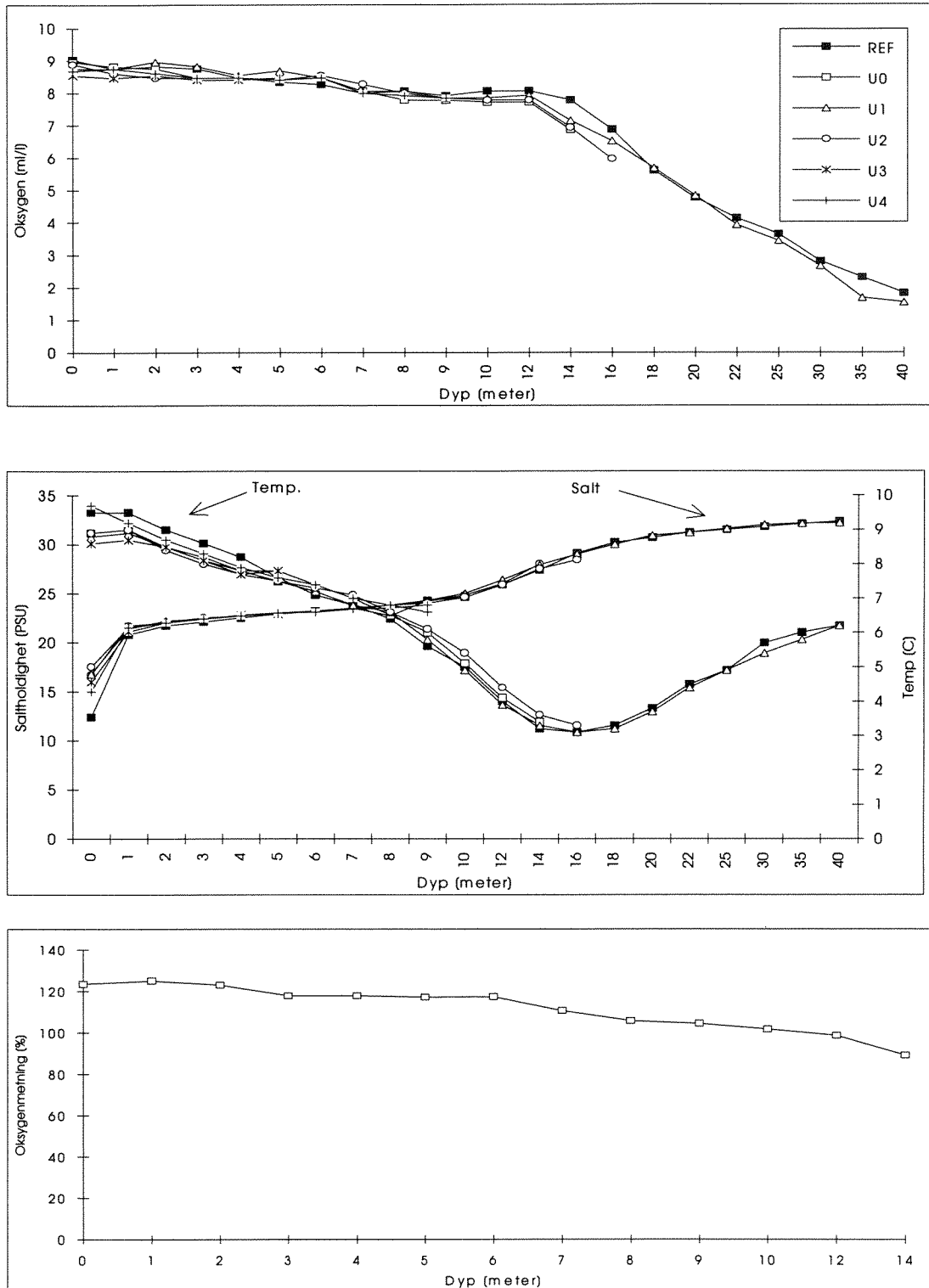
Figur 5: Oksygeninnhold, saltholdighet og temperatur den 06.05.1994. Oksygenmetning i stasjon Uo.
