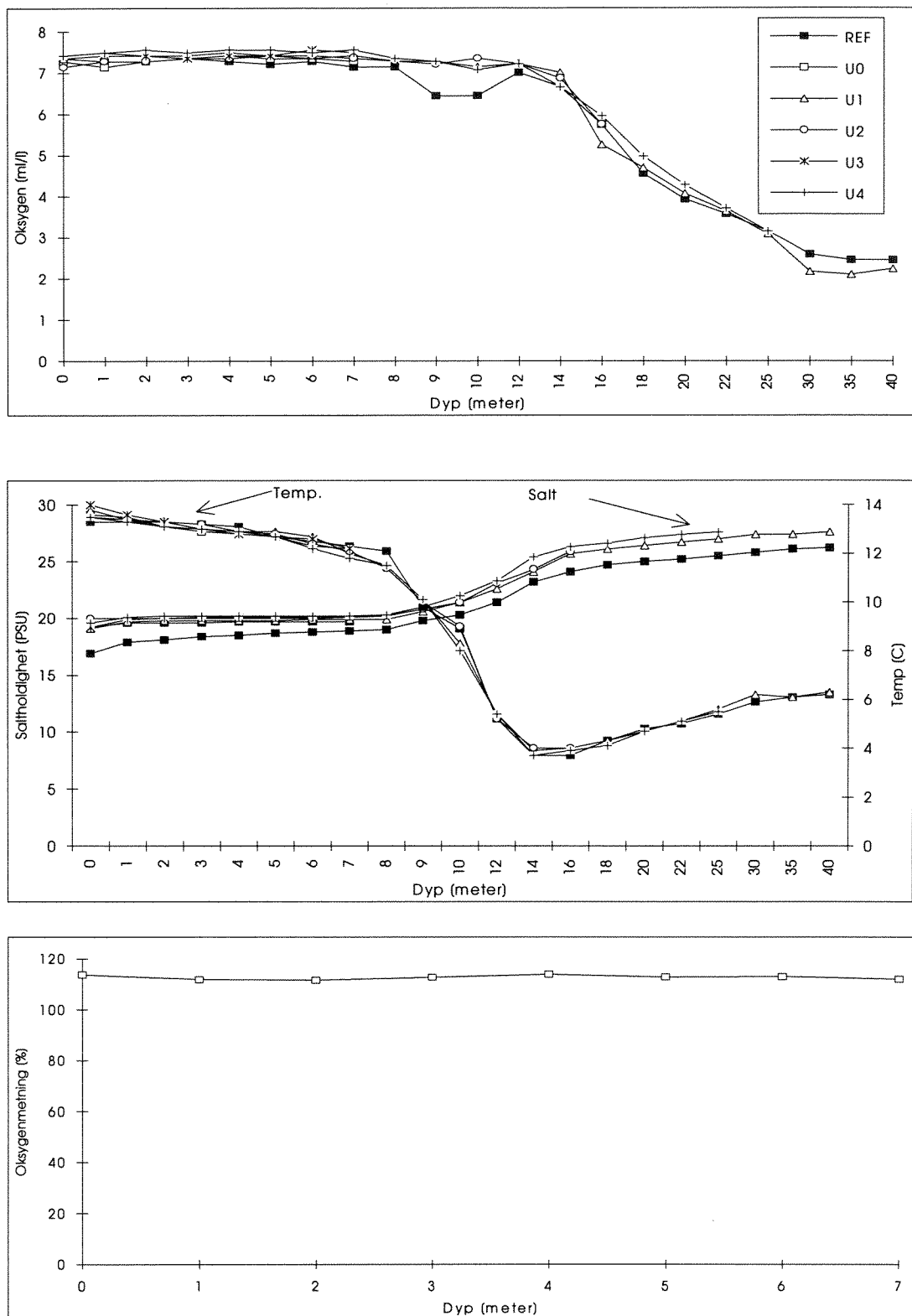
Figur 8: Oksygeninnhold, saltholdighet og temperatur den 06.06.1994. Oksygenmetning i stasjon U0.
