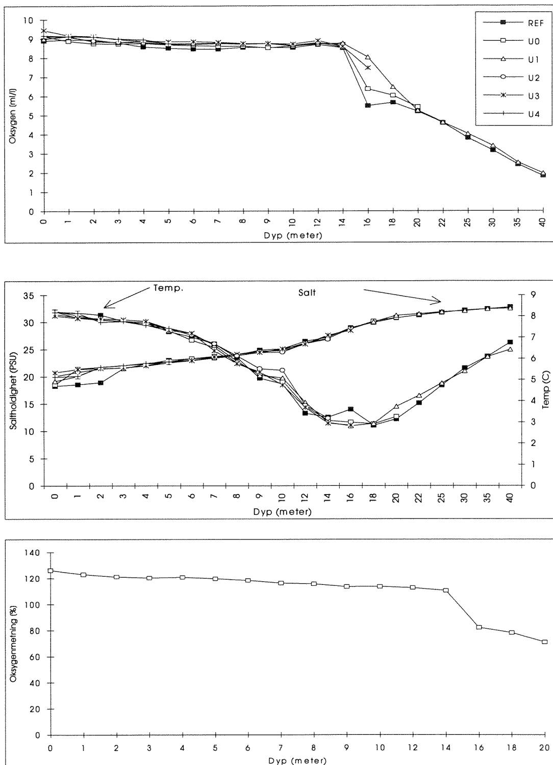
Figur 4: Oksygeninnhold, saltholdighet og temperatur den 29.04.1994. Oksygenmetning i stasjon Uo.
