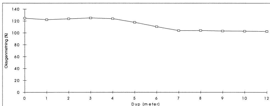
Figur 6: Oksygeninnhold, saltholdighet og temperatur den 24.05.1994. Oksygenmetning i stasjon Uo.
