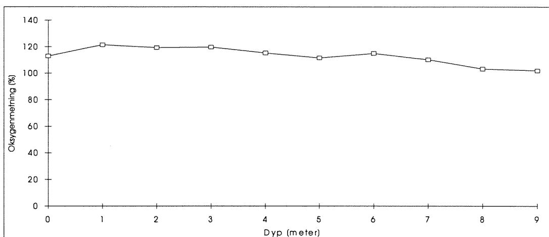
Figur 7: Oksygeninnhold, saltholdighet og temperatur den 30.05.1994. Oksygenmetning i stasjon U0.
