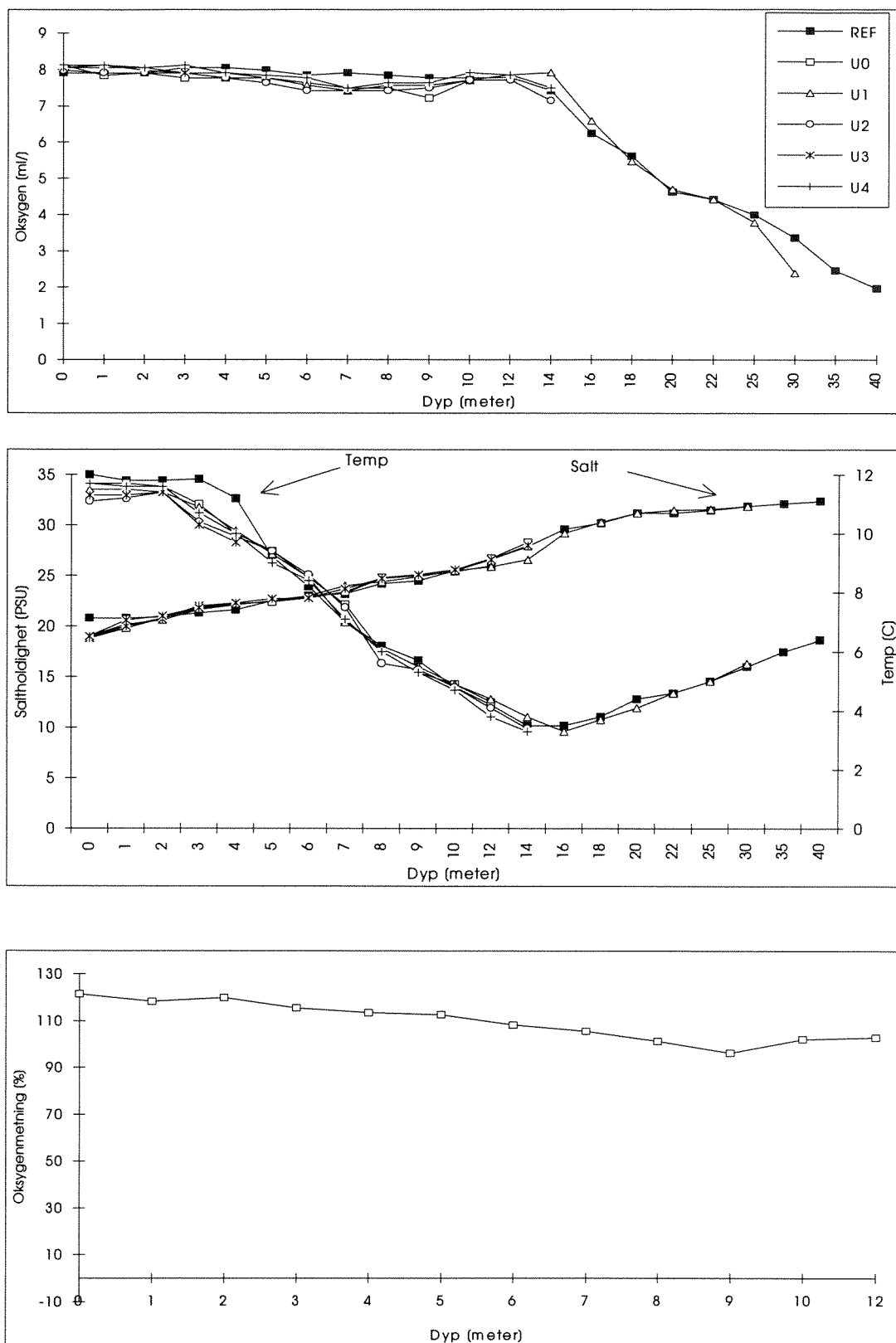
Figur 10: Oksygeninnhold, saltholdighet og temperatur den 20.06.1994. Oksygenmetning i stasjon Uo.
