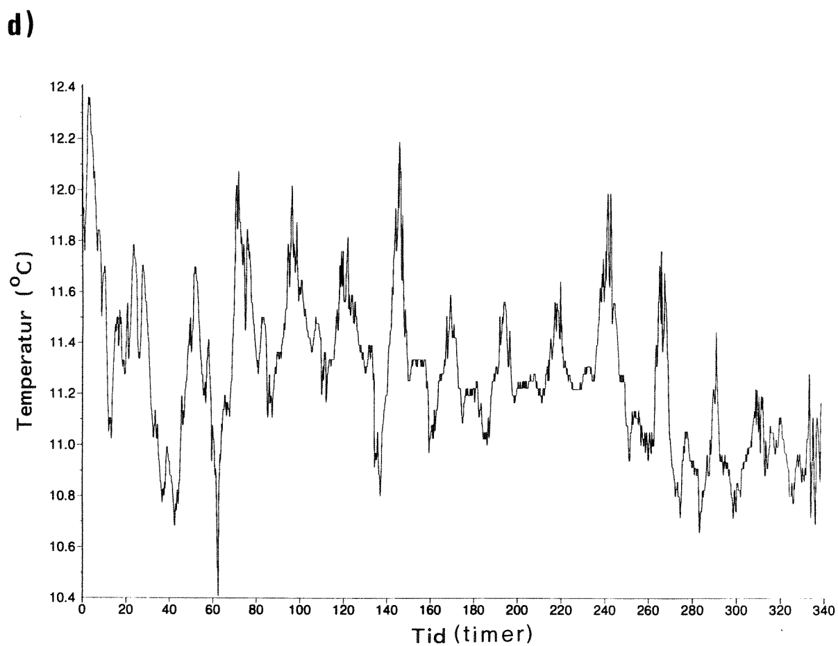
Fig. 3.2. Resultater av målinger på 2,5 meters dyp for perioden 14.-29.09.93 på stasjon A1 (ved fersk-vannsutslippet) med angivelse av a) strømhastighet, b) strømreretning, c) nettostrøm og d) temperatur.
