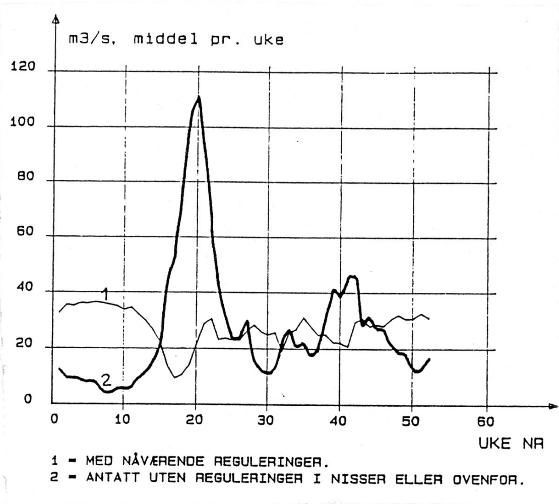
Figur 4. Midlere vannføring ut av Nisser ved reguleringer pr. 1989 (kurve 1). Antatt vannføring uten regulering i Nisser eller ovenfor (kurve 2). (Fra Arendals Vasdrags Brugseierforening 1989).
