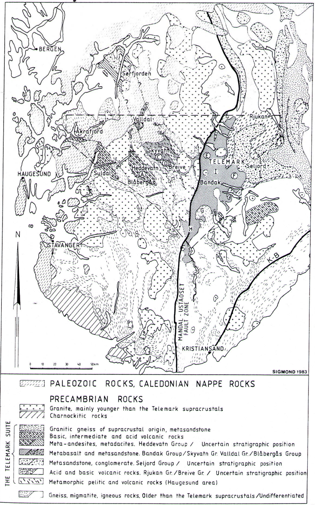
Figur 2. Geologisk kart over den sørlige delen av Norge (Fra Maijer og Padget 1987).
