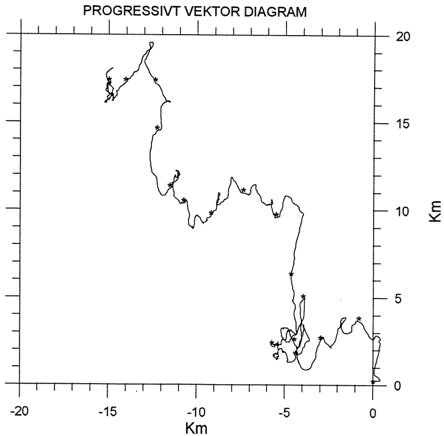
Figur V2. Strømmålingane i 4 m djup ved Trellevik fordelt i retningssektorar, samt progressiv vektor diagram for målingane.
