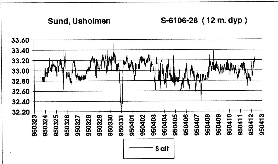
Figur 3.2a. Målt sjøtemperatur og salinitet i 12 m djup ved Usholmen i perioden 23. mars - 13. april 1995.
