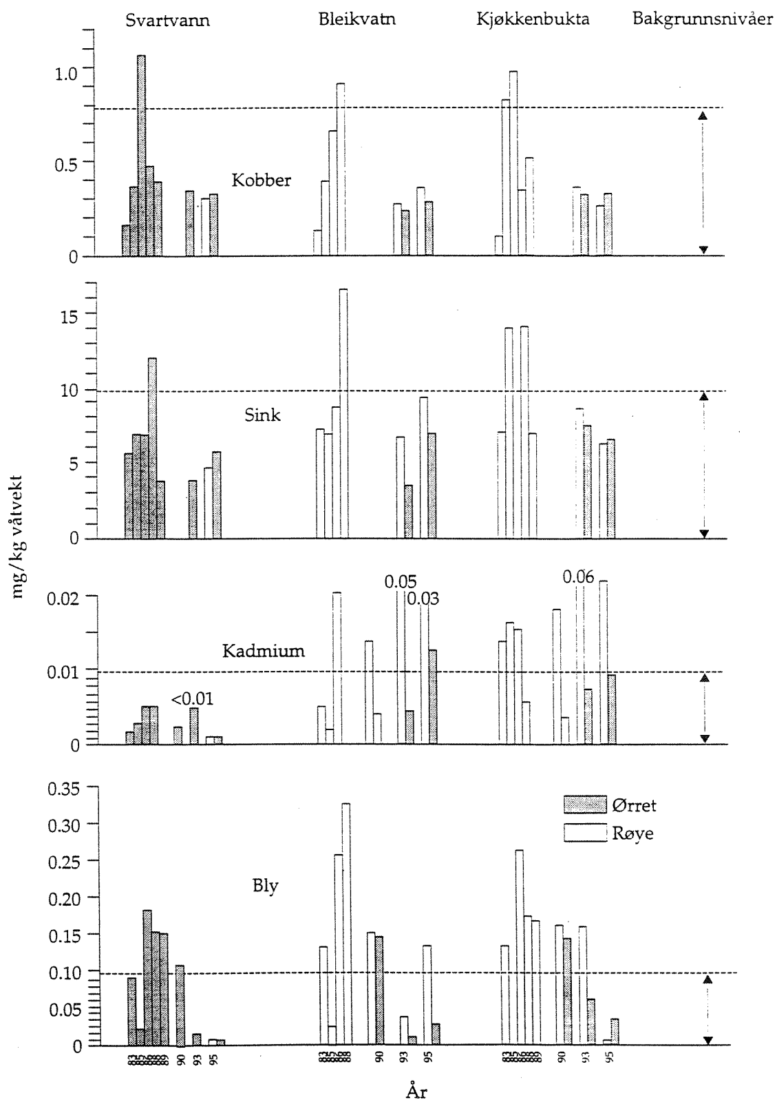
Figur 9. Tungmetaller i filét (muskulatur) av ørret og røye fra Bleikvatn, Kjøkkenbukta og Svartvatn. Middelerdier 1983, 85, 86, 88, 91, 93 og 95. Mg/kg våtvekt. Over stiptet strek: høyere enn bakgrunn.
