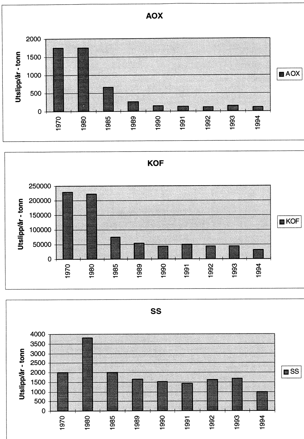
Fig. 4.4. Borregaard Industries Ltd. Utslipp av klororganiske forbindelser (AOX), oppløst organisk materiale (KOF) og suspendert stoff (SS) i årene 1970, 1980, 1985 og 1989-1994(tonn/år).
