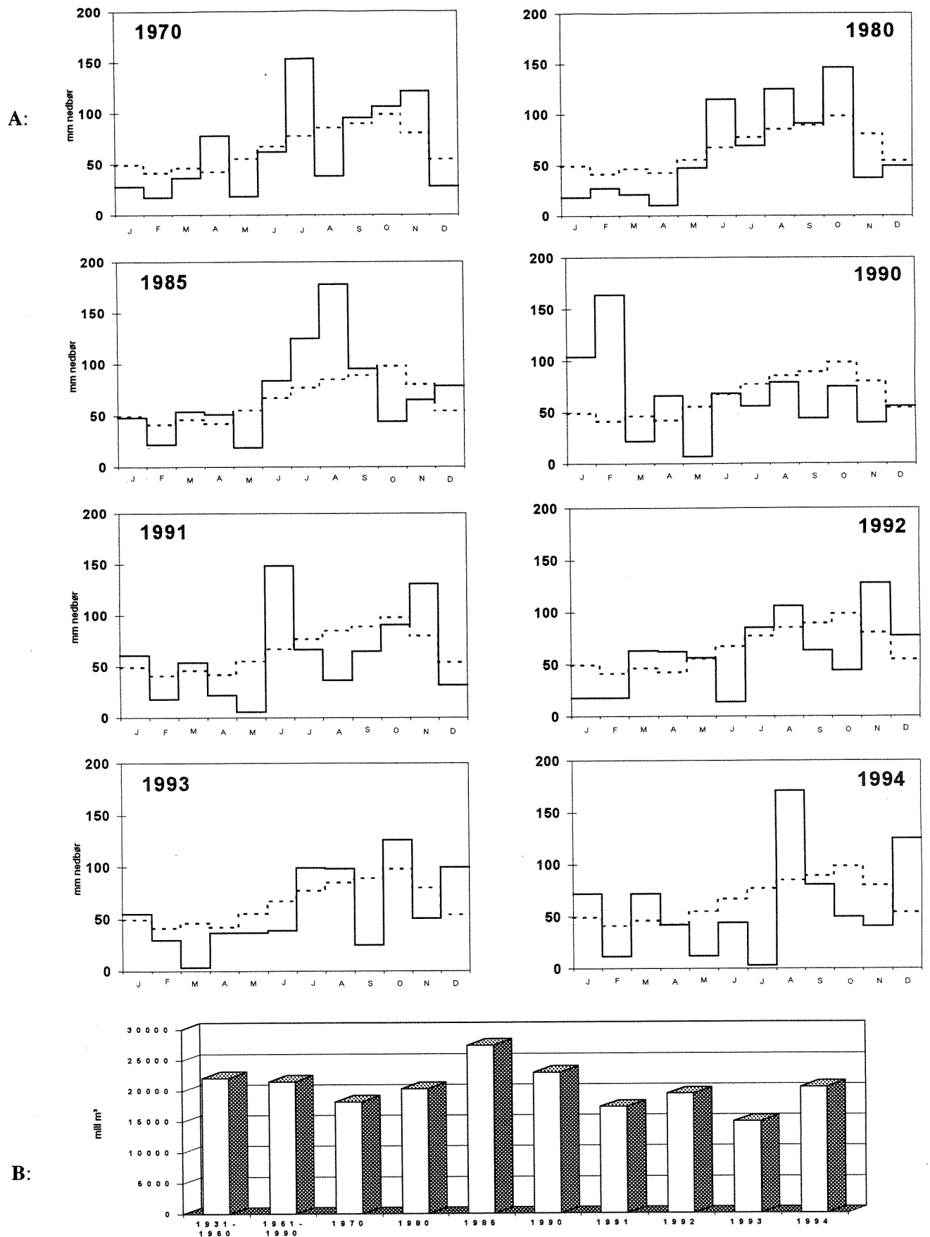
Fig. 3.9. Nedbør.
