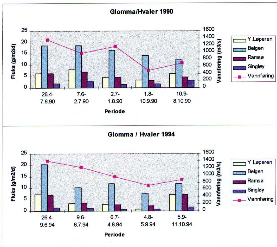
Figur 18. Fluks av partikulært materiale ( \text{g/m}^2/\text{d} ) i fem perioder fra 26.4 - 8.10.90 og 11.10.94. Samt vannføring målt ved Sarpfoss ( \text{m}^3/\text{s} ) i de samme periodene.
