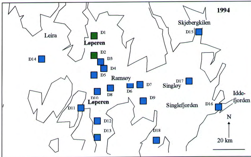
Figur 25. Klassifisering av tilstanden på de 18 bløtbunnfaunastasjonene i 1994. Graden av påvirkning varierte fra moderat (grønn farge) i dyppartier i indre Løperen, til liten (blå) i midtre og ytre områder. Klassifisering er foretatt etter Rygg og Thélin, 1993.
