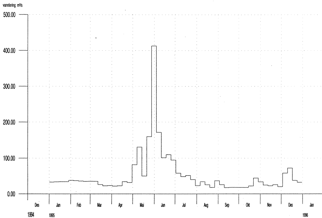
Figur 4. Karakteristiske 7-døgns vannføringer i Orkla ved Syrstad i 1995.
