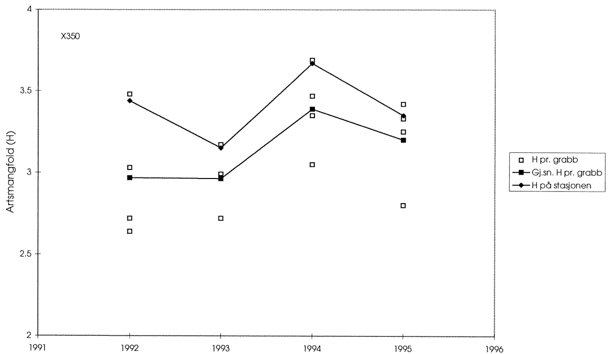
Figur 40. Artsmangfold (H) på stasjon X350 i 1990-1995.
