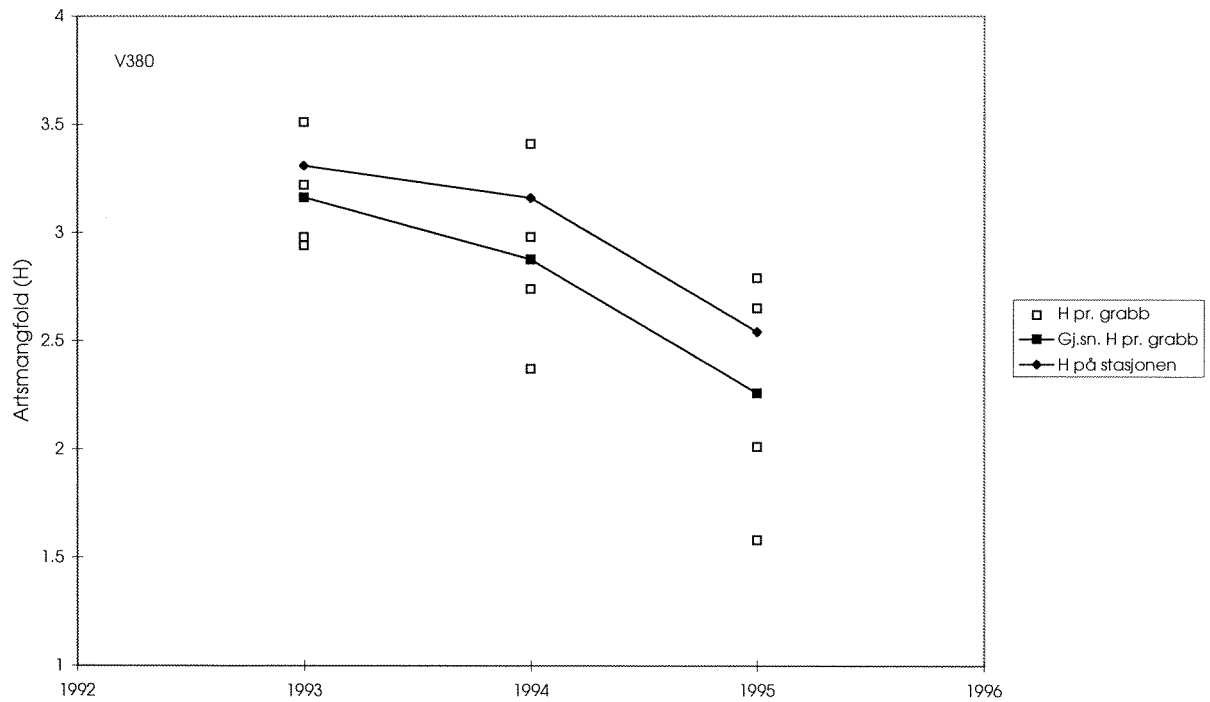
Figur 38. Artsmangfold (H) på stasjon V380 i 1990-1995.
