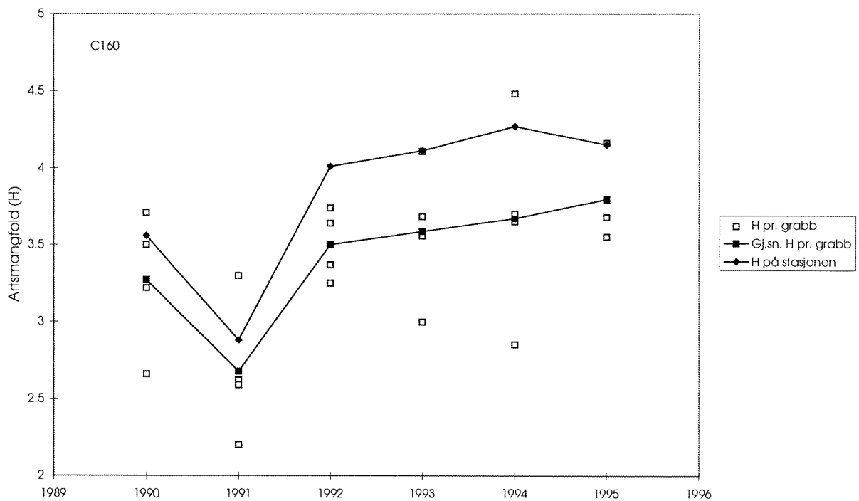
Figur 30. Artsmangfold (H) på stasjon C160 i 1990-1995.
