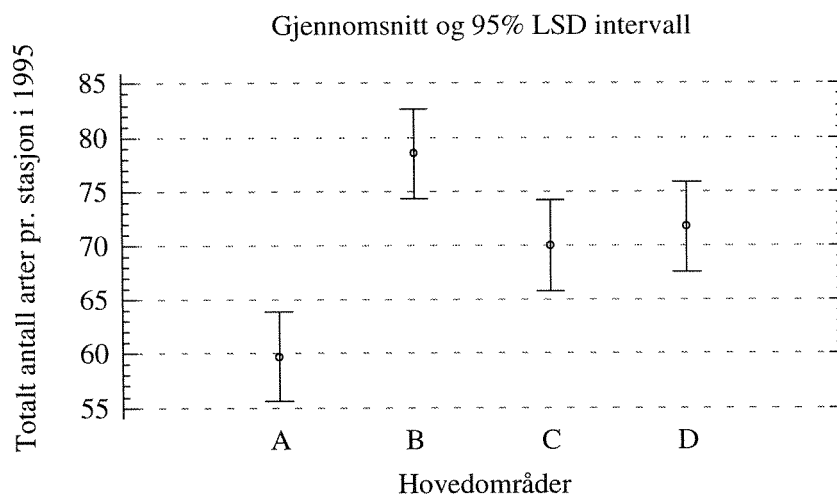
Figur 57. Gjennomsnitt av total antall arter registrert pr.stasjon i 1995 innen hvert av hovedområdene. LSD (Least Significant Difference) er parvise t-tester mellom gj.sn.-verdier for faktorene
