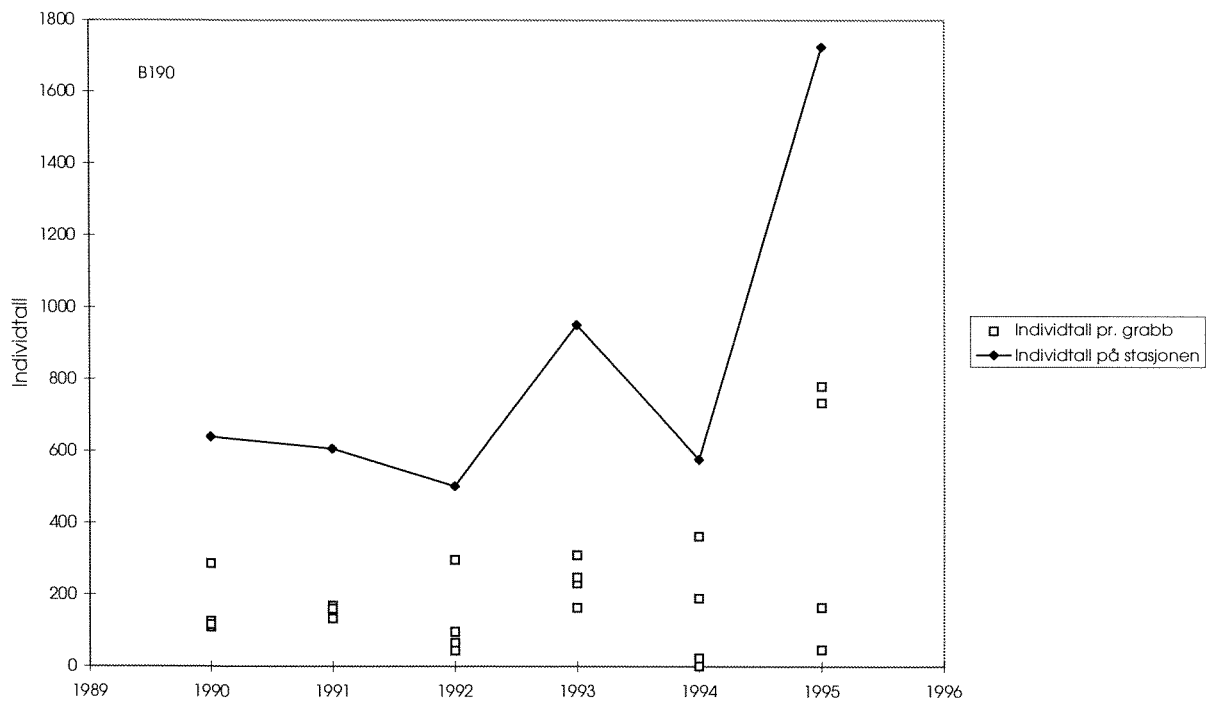
Figur 23. Individtall på stasjon B190 i 1990-1995.
