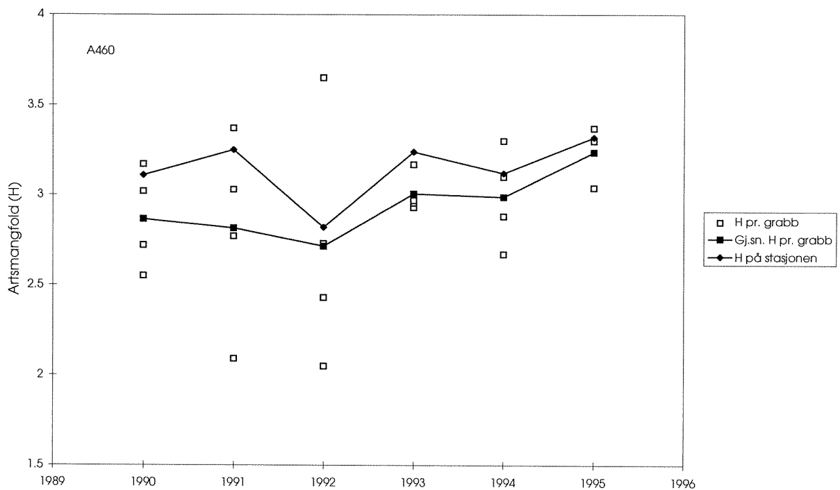
Figur 16. Artsmangfold (H) på stasjon A460 i 1990-1995.
