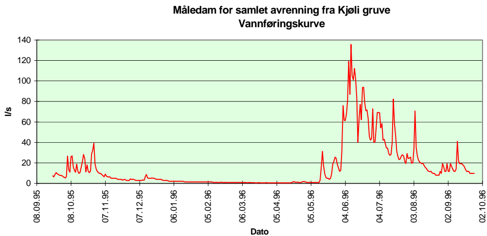
Figur 4. Døgnmiddelvannføringer ved st.1 Måledam for samlet avrenning fra Kjøli gruve.
